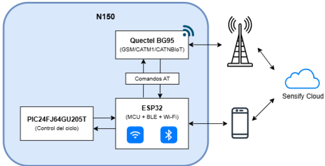
FIGURA 2.2. Arquitectura de conectividad del controlador N150.
