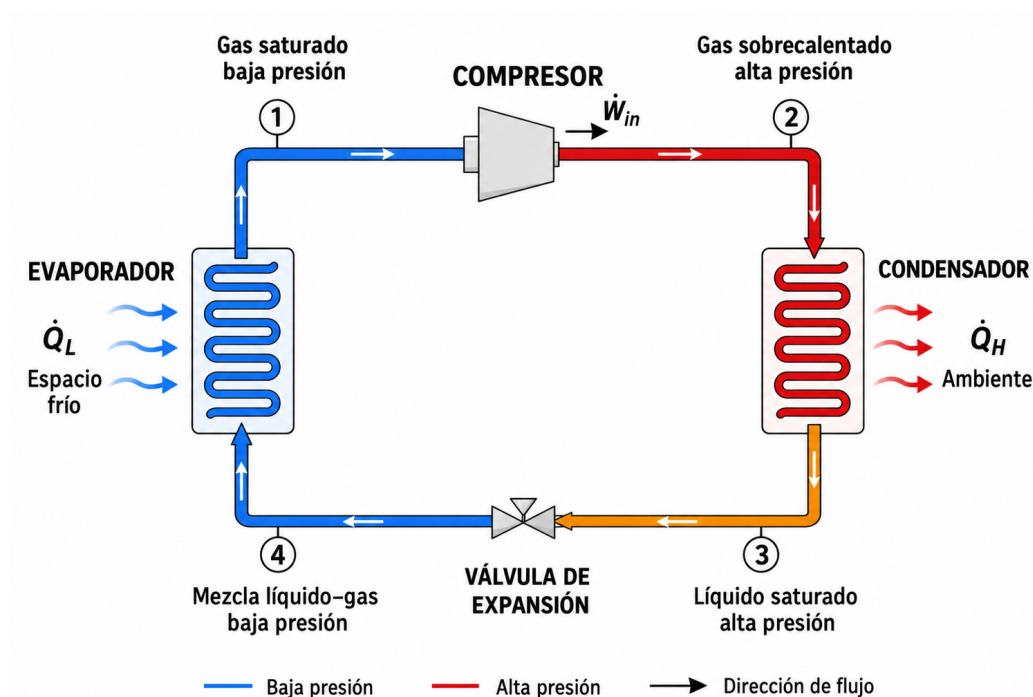
FIGURA 2.1. Esquema del ciclo de refrigeración: compresor, condensador, dispositivo de expansión y evaporador.
