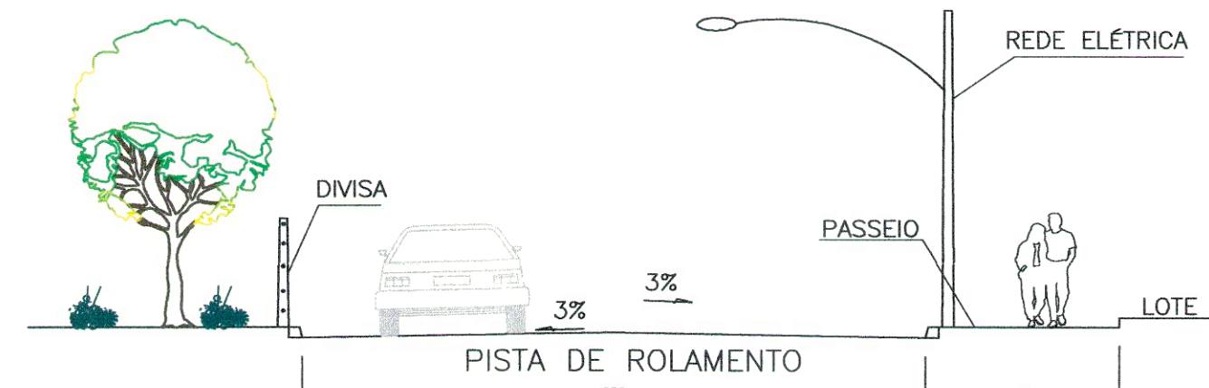
SEÇÃO TRANSVERSAL - RUAS 10.00m RUA JL 1, JL 14, JL 15
