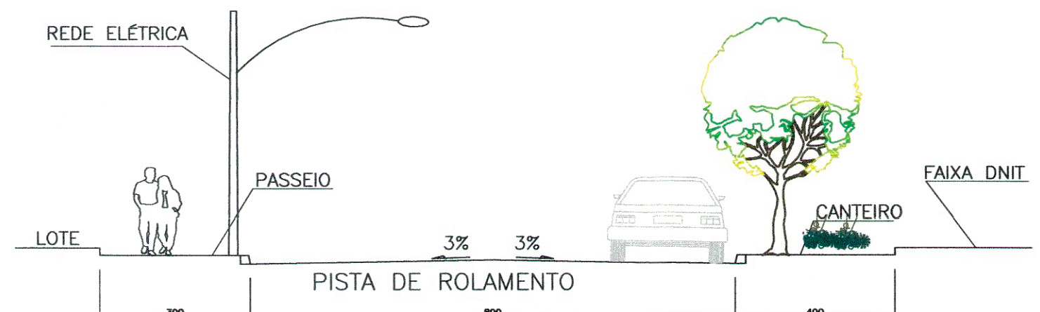
SEÇÃO TRANSVERSAL - RUAS 15.00m RUA JL 17
