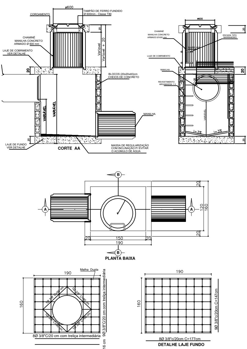
POÇO DE VISITA COM DEGRAU
