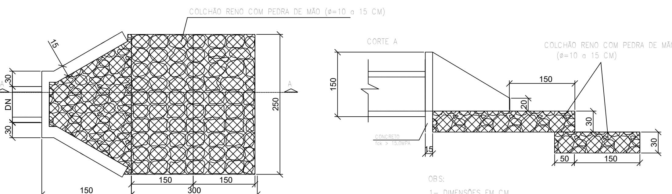
ALA DE REDE TUBULAR DISSIPADOR DE ENERGIA
