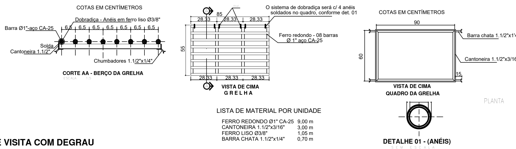
POÇO DE VISITA COM DEGRAU
