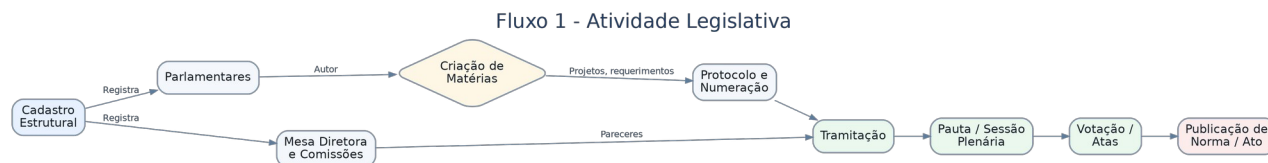
Figura 2 - Diagrama do fluxo: Fluxo de Atividade Legislativa.
