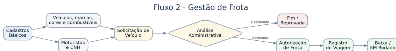
Figura 3 - Diagrama do fluxo: Fluxo de Gestão de Frota.
