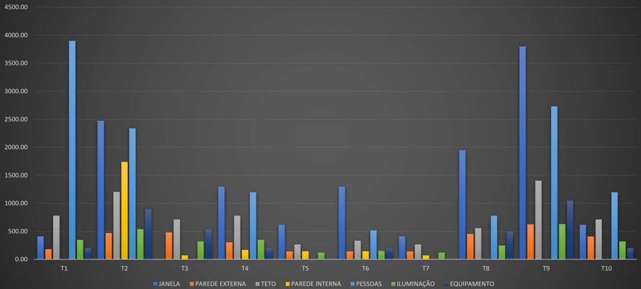
CARGA TÉRMICA POR AMBIENTE
