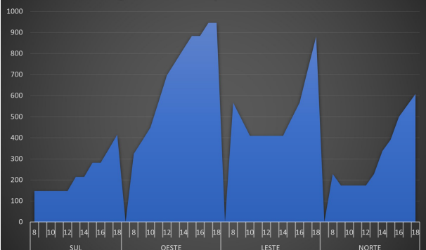
Carga térmica de paredes externas.
