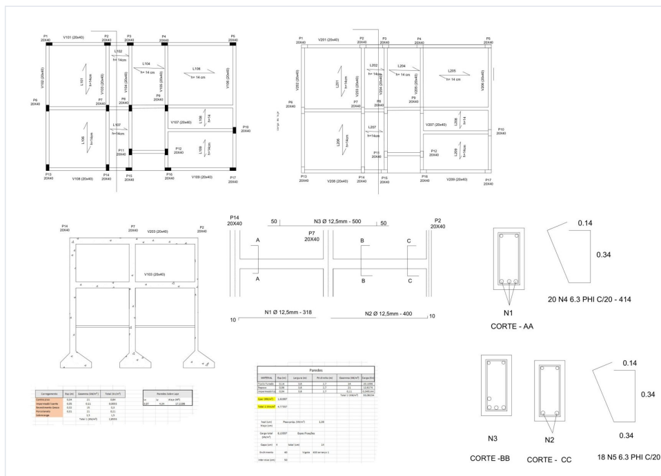
Planta de fôrmas com pilares e vigas 20×40 e lajes h = 14 cm, mais o detalhamento de armaduras das vigas (cortes AA, BB e CC). PDF da prancha
