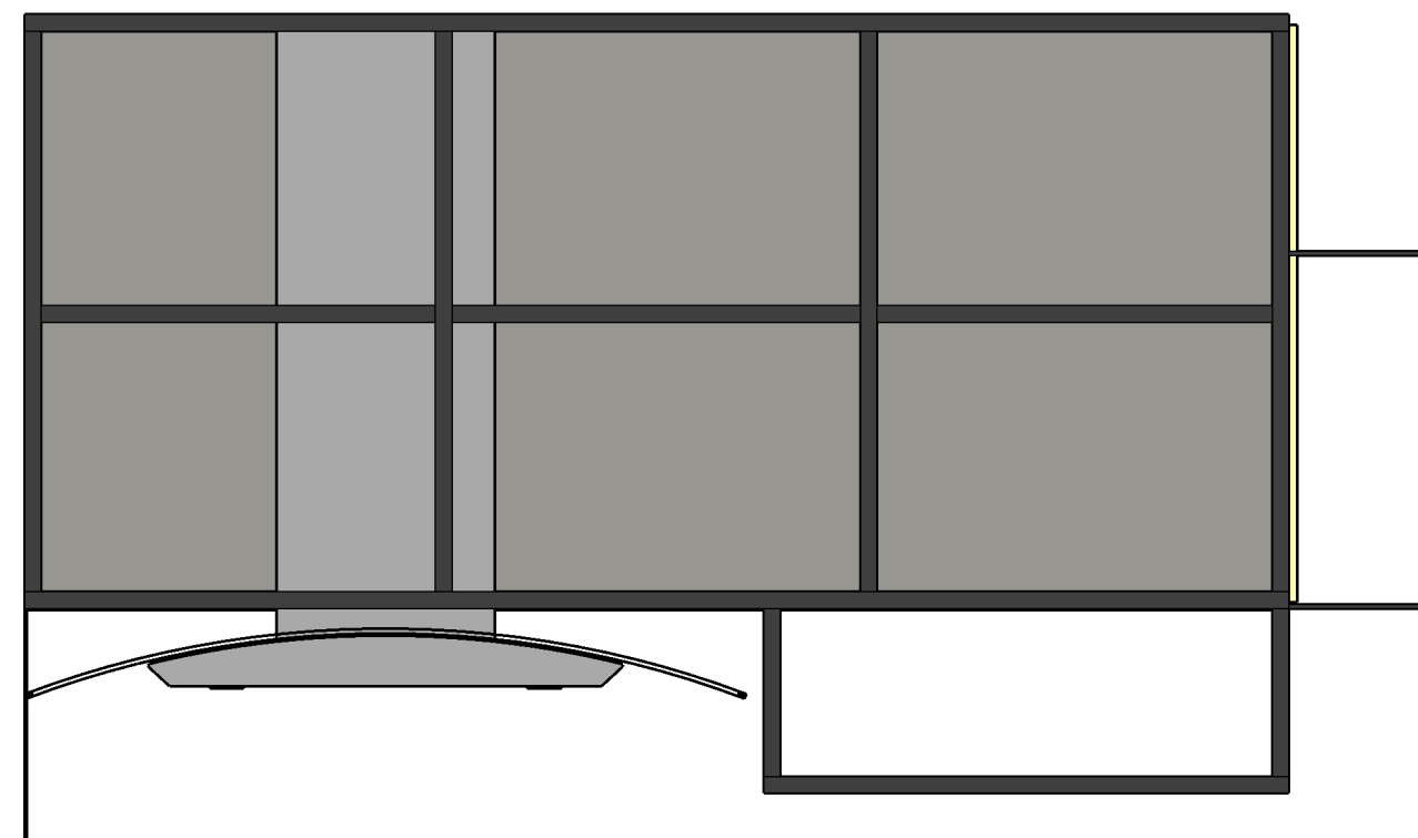
2 VISTA 2 1:10
