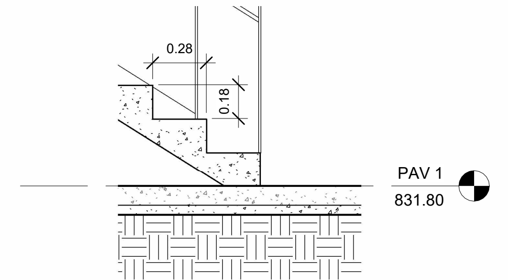
3 DETALHE - ESCADA 1 : 20
