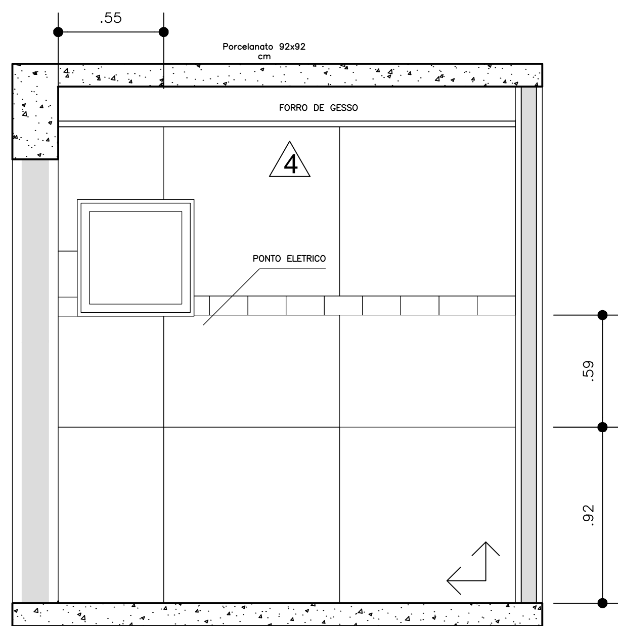
1 ELEVACÃO 4 ESCALA: 1:50
