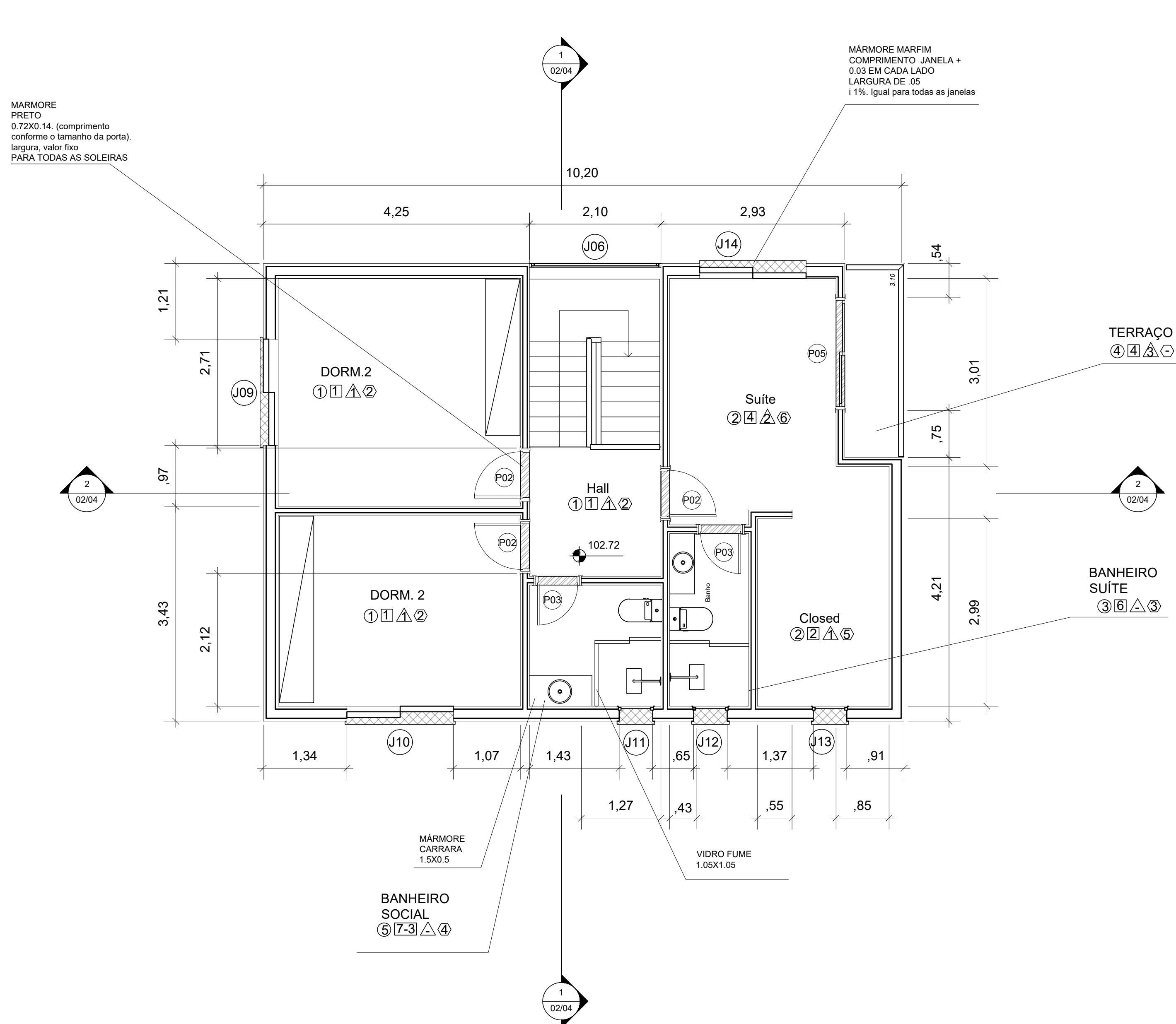
2 PLANTA PAV. SUPERIOR ESCALA: 1:50
