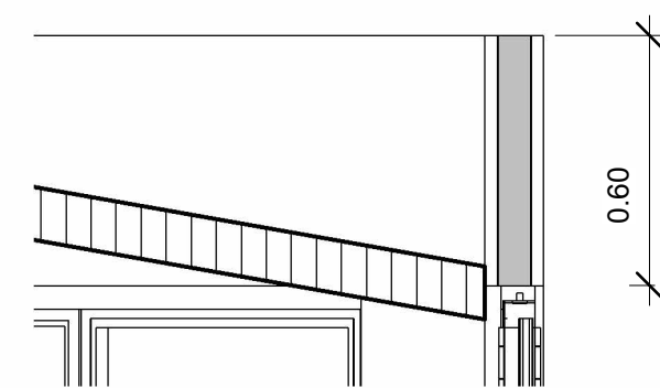
5 DETALHE - COBERTURA 1 : 20
