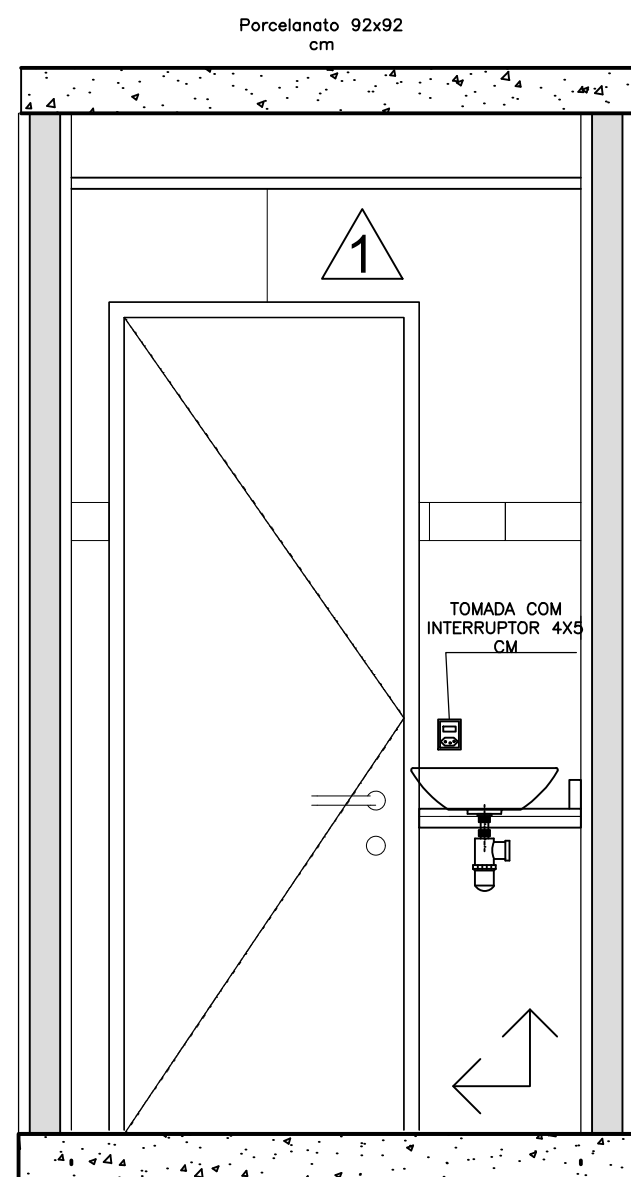
2 ELEVACÃO 1 ESCALA: 1:20
