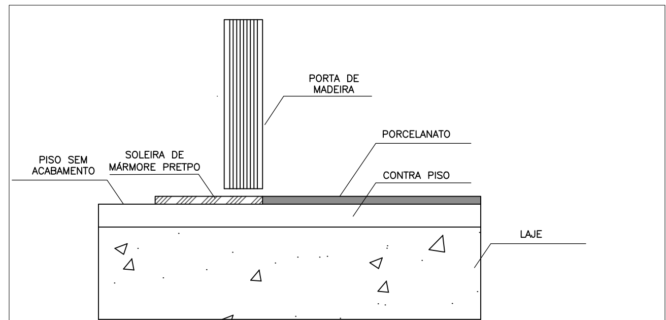
2 ELEVACÃO 1 ESCALA: 1:20
