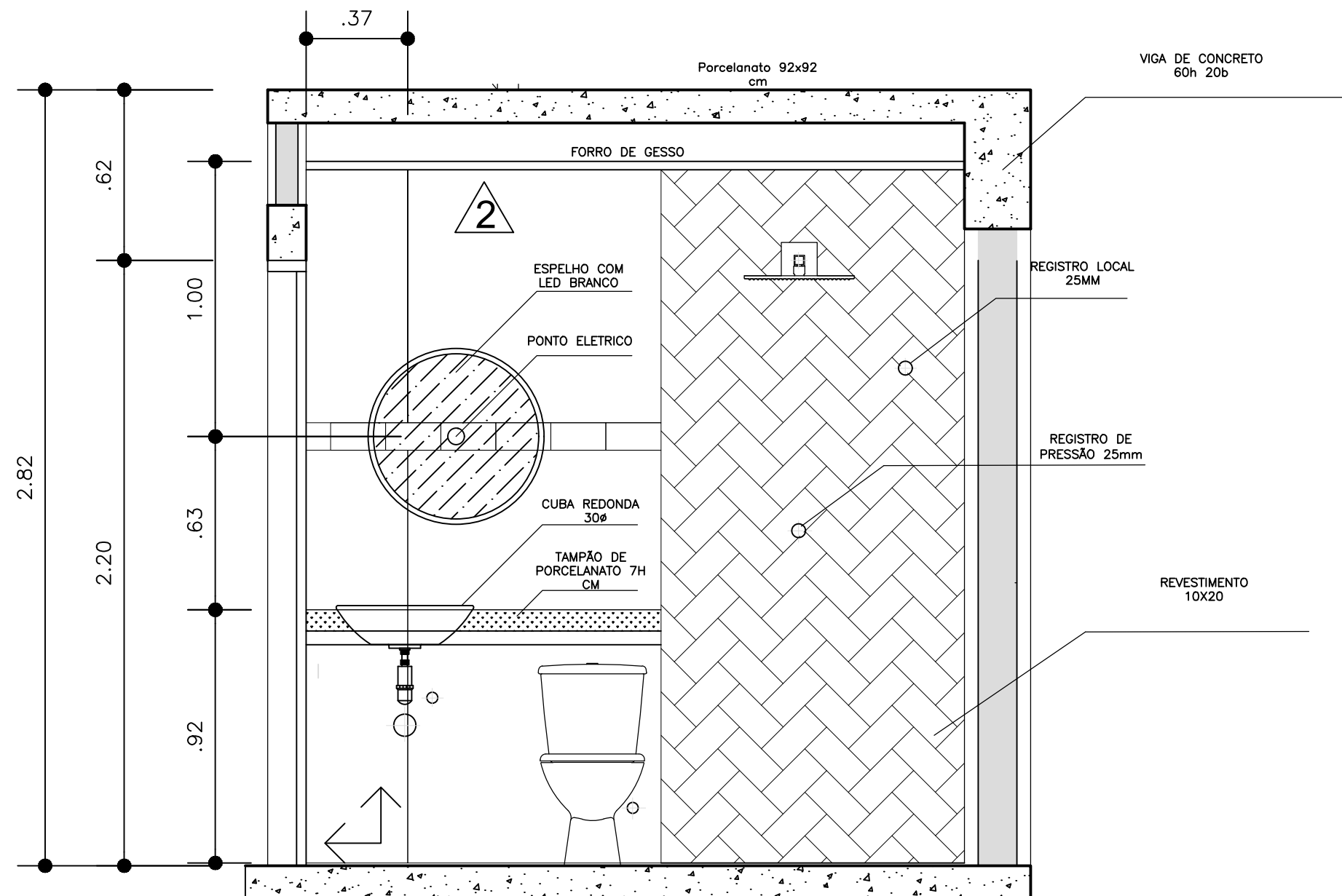
3 ELEVACÃO 2 ESCALA: 1:20
