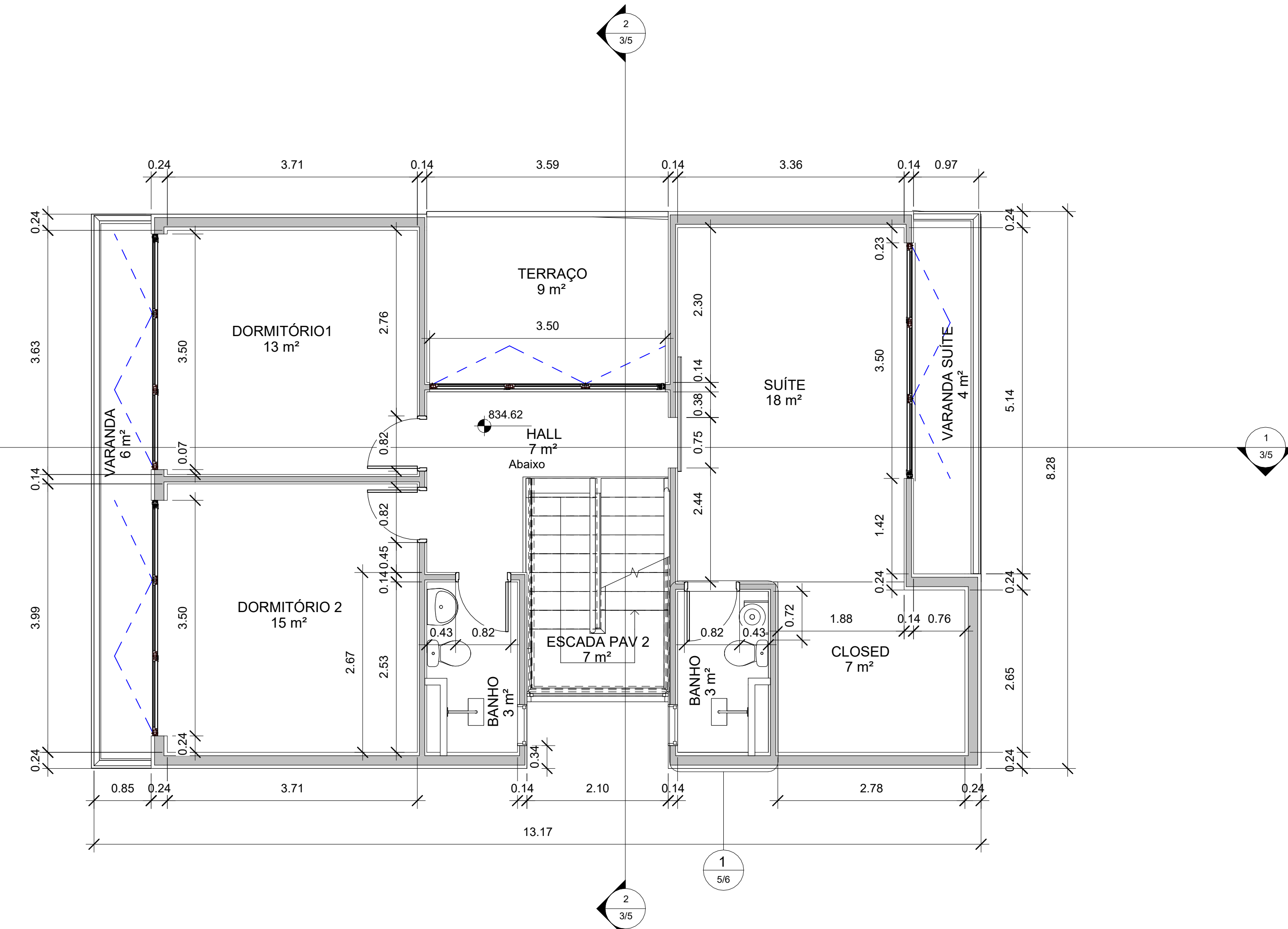
2 PAV 2 1 : 50
