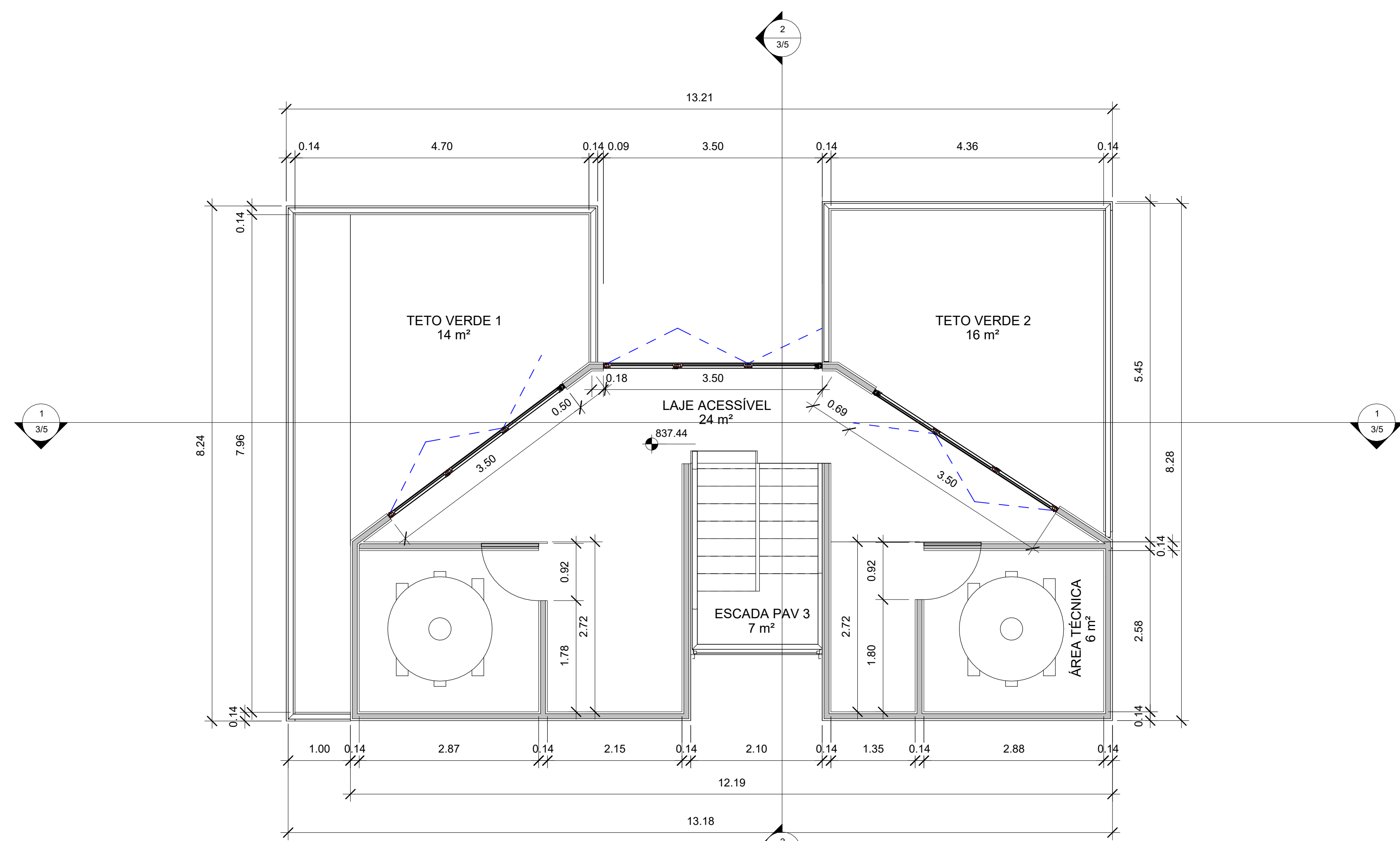
3 PAV 3 1 : 50
