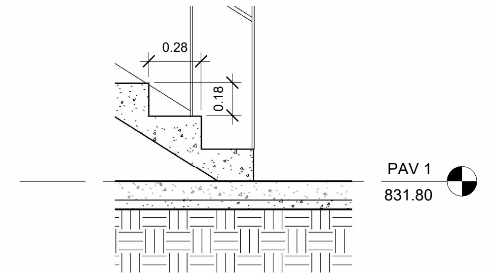
3 DETALHE - ESCADA 1 : 20
