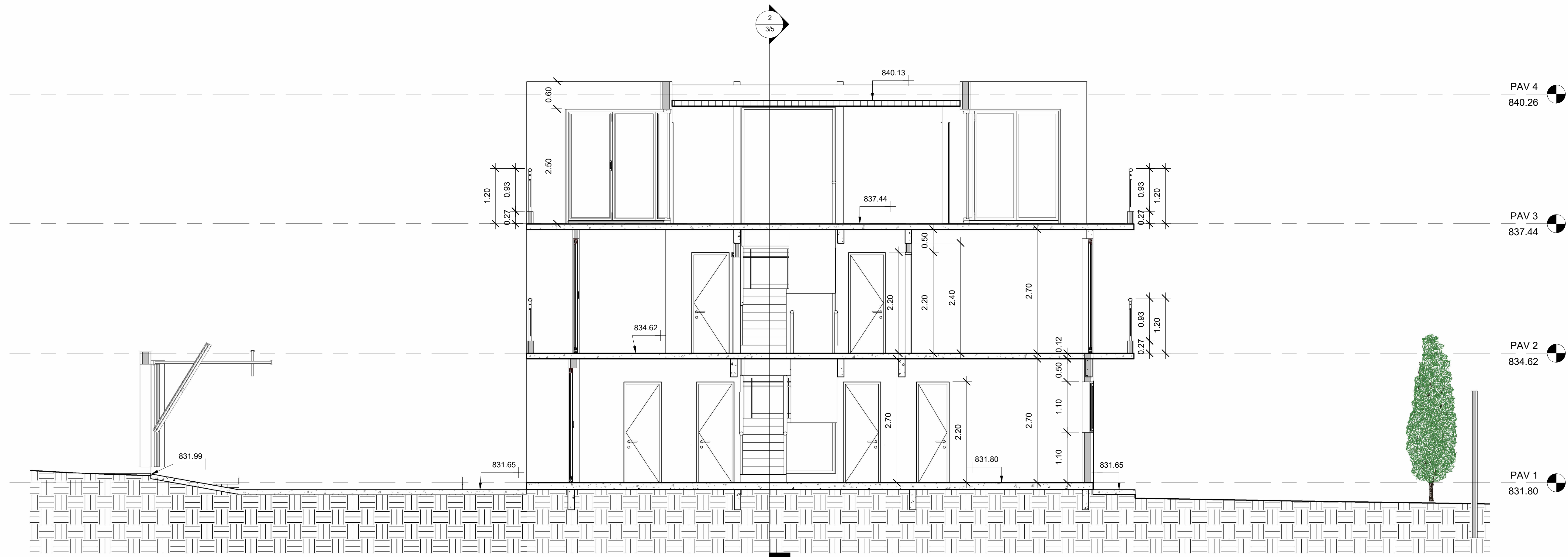
1 CORTE LONGITUDINAL 1 : 50
