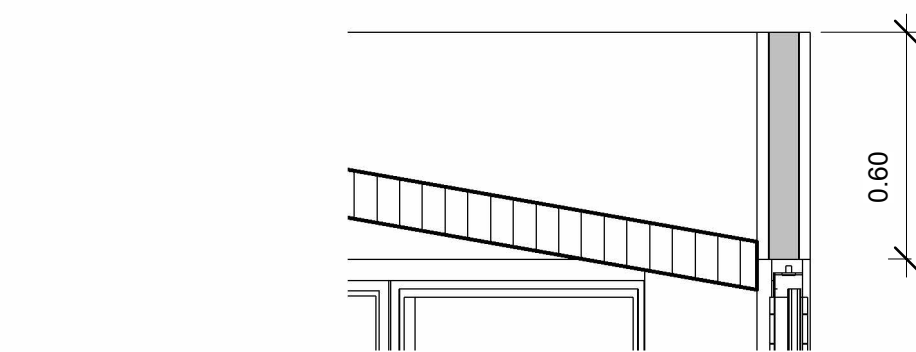
5 DETALHE - COBERTURA 1 : 20
