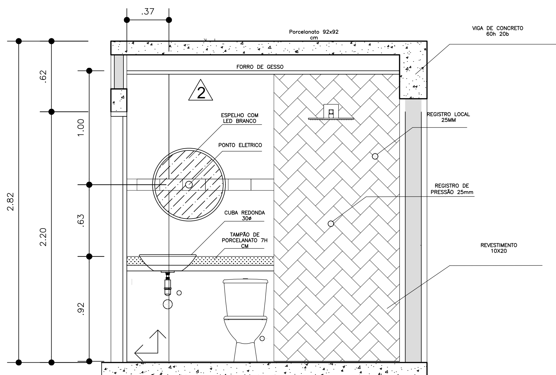
3 ELEVÇÃO 2 ESCALA: 1:20
