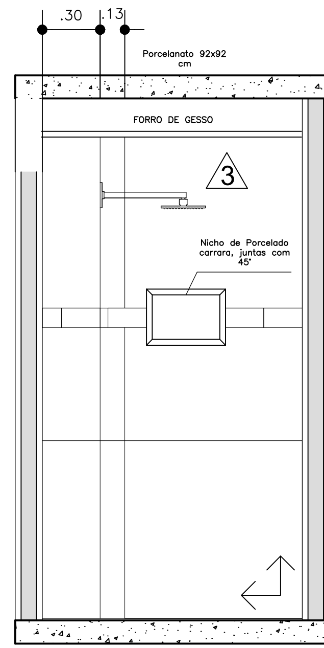
4 ELEVÇÃO 3 ESCALA: 1:20
