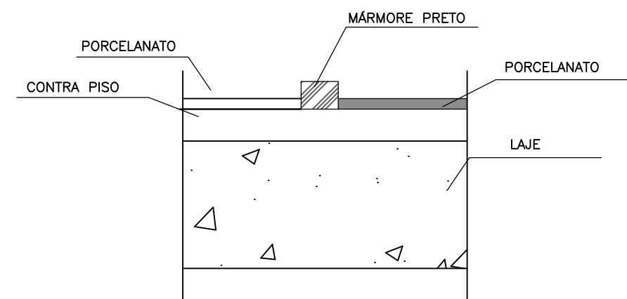
2 ELEVÇÃO 1 ESCALA: 1:20
