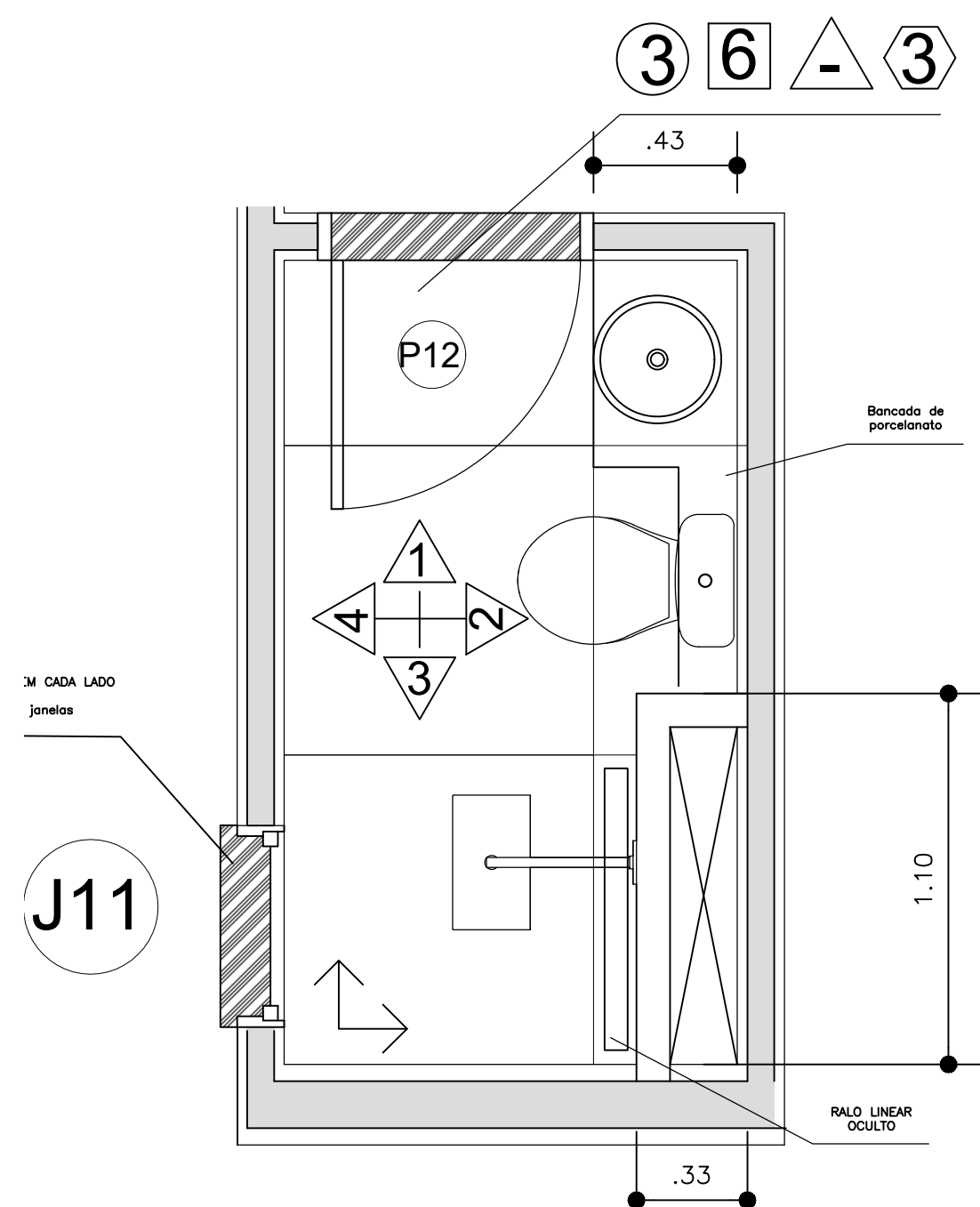
1 BANHEIRO DA SUÍTE ESCALA: 1:20
