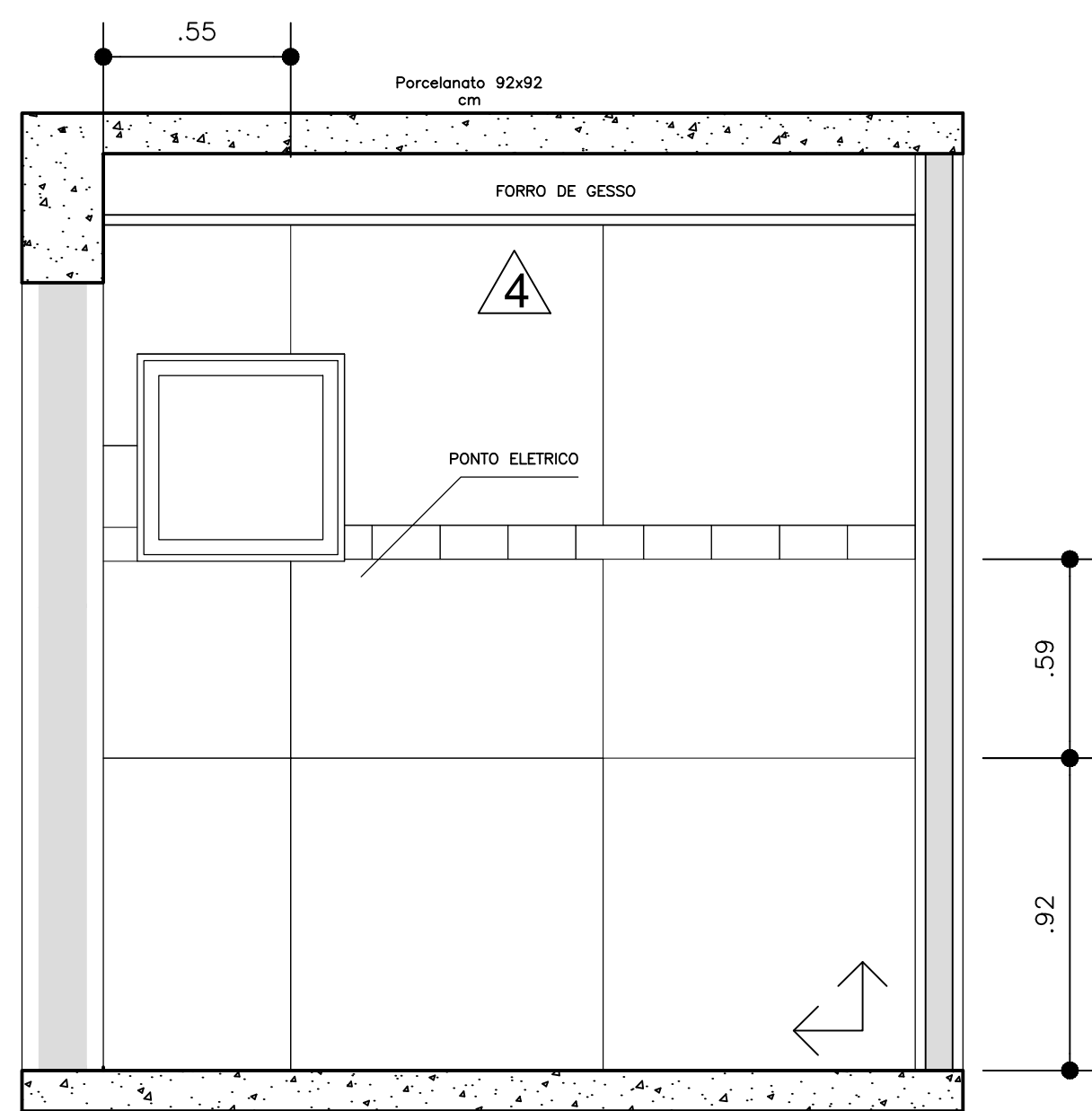
1 ELEVÇÃO 4 ESCALA: 1:50
