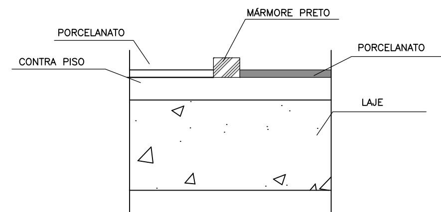
2 ELEVÇÃO 1 ESCALA: 1:20
