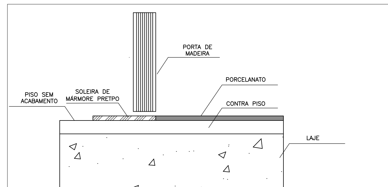
2 ELEVÇÃO 1 ESCALA: 1:20
