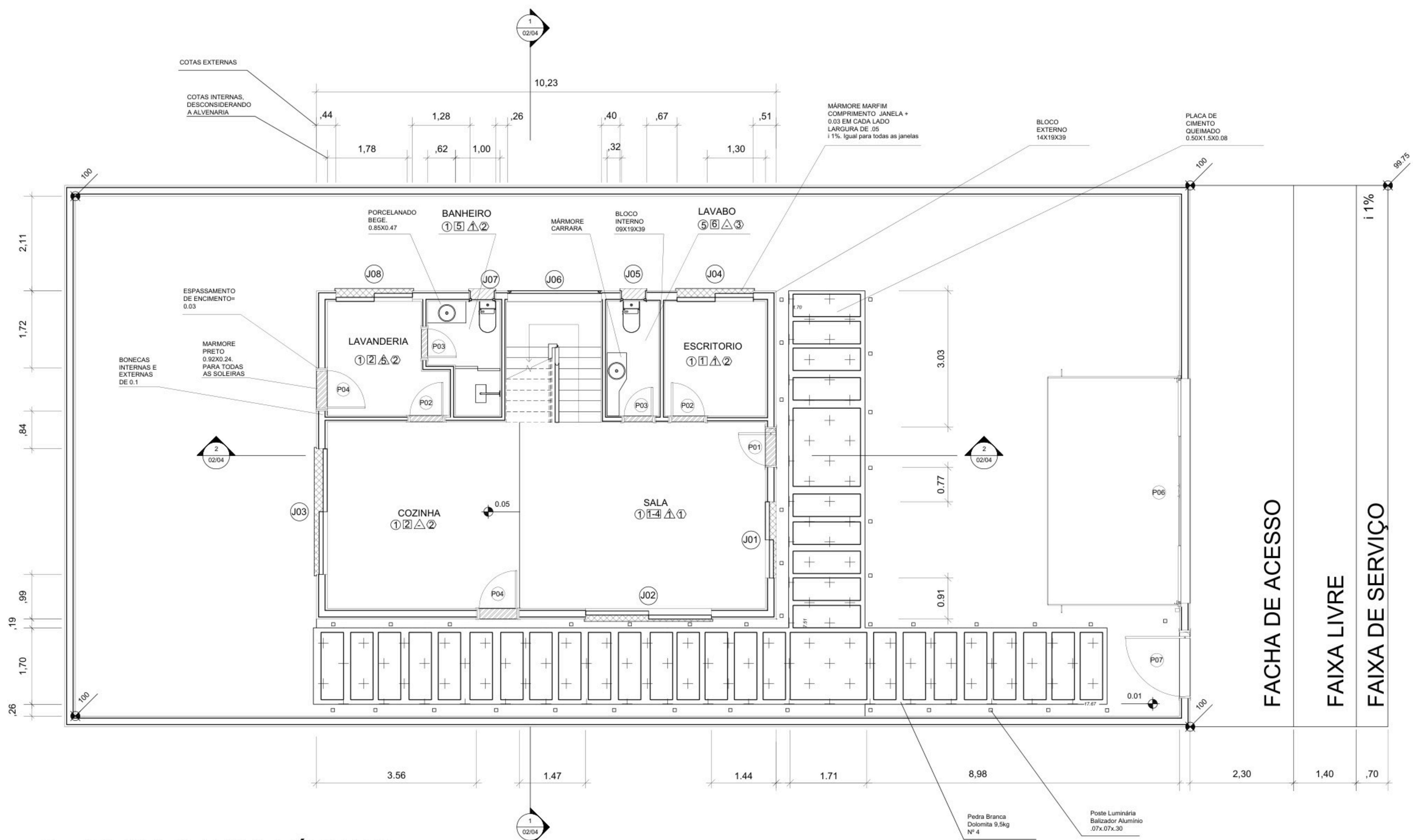
1 PLANTA PAV. TÉRREO ESCALA: 1:50
