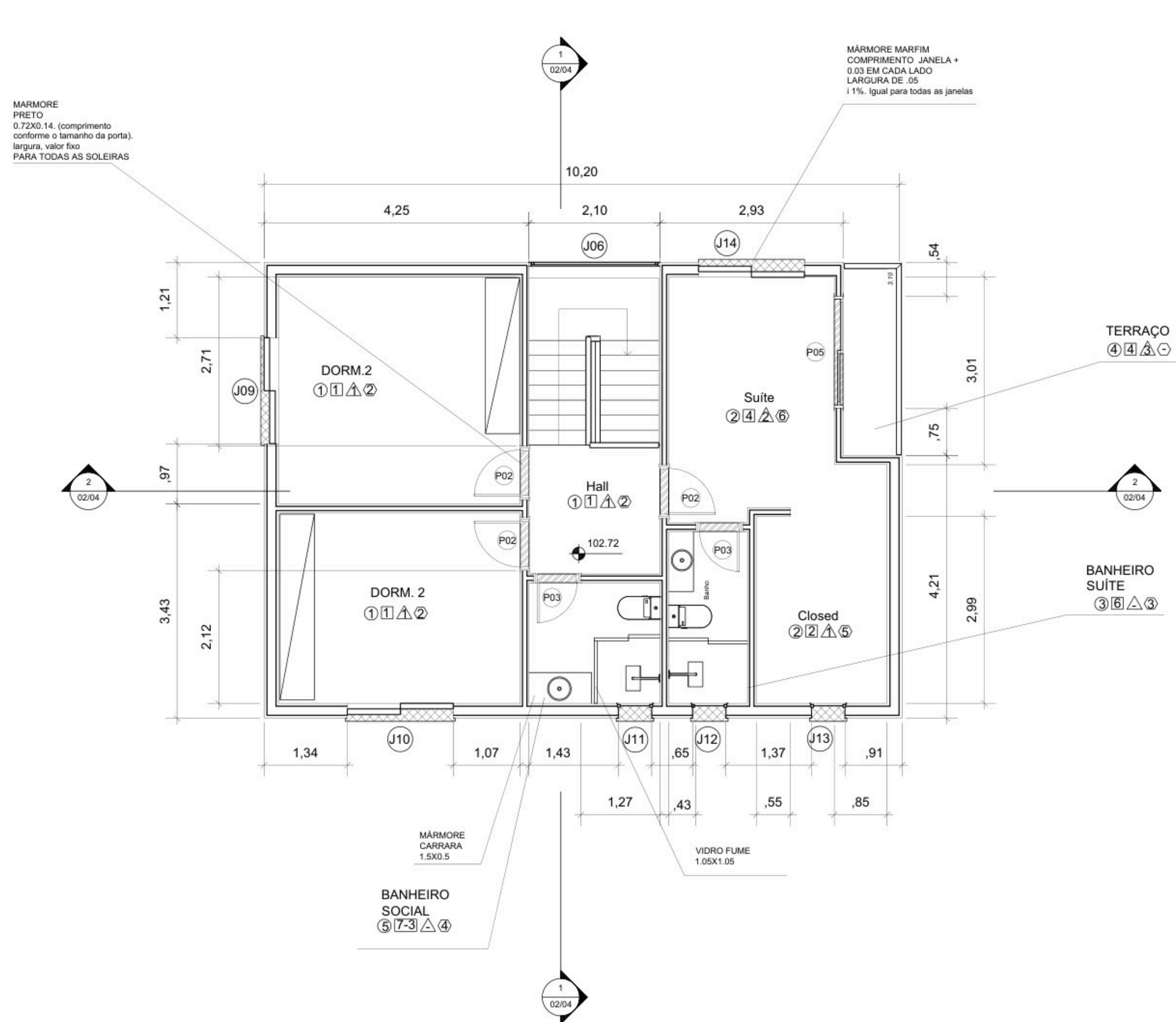
2 PLANTA PAV. SUPERIOR ESCALA: 1:50
