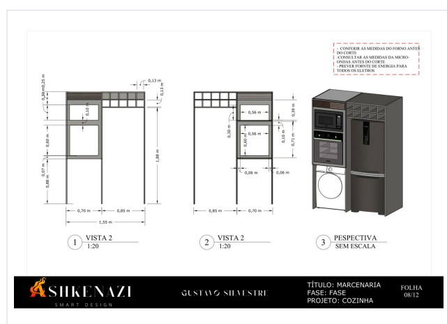
Folha 08: marcenaria da torre quente
