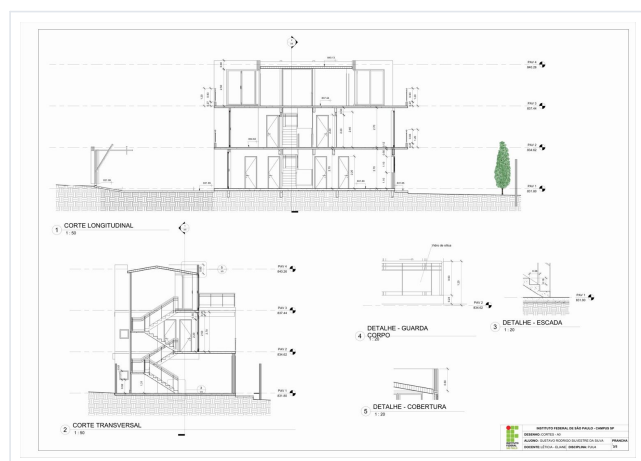
Cortes e detalhes
