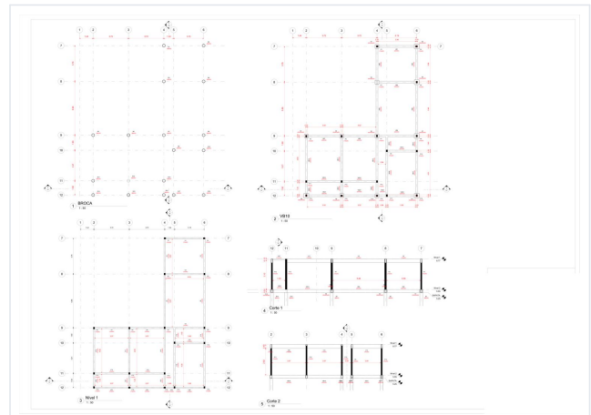
Fundações, baldramas, pilares e vigas
