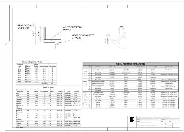
Folha 04: detalhes e tabelas
