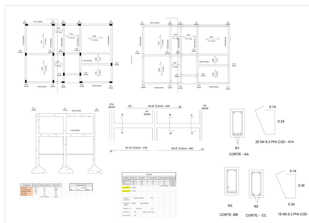
Estrutura e armaduras
