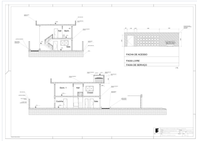
Folha 02: cortes e gradil
