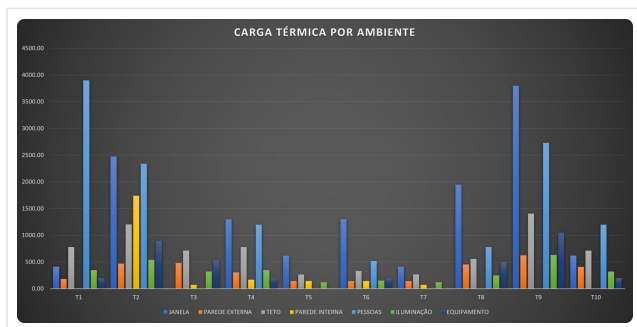
Carga térmica por ambiente e por fonte
