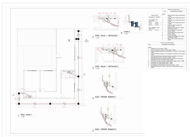
Esgoto sanitário: planta, detalhes e isométricos
