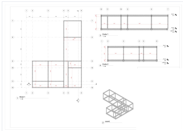
Concepção estrutural: planta, cortes e 3D
