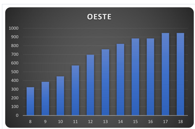
Variação horária da carga: fachada oeste
