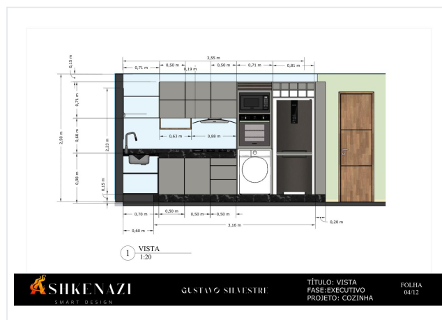
Folha 04: vista cotada 1:20
