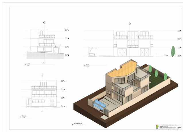
Fachadas e isométrica
