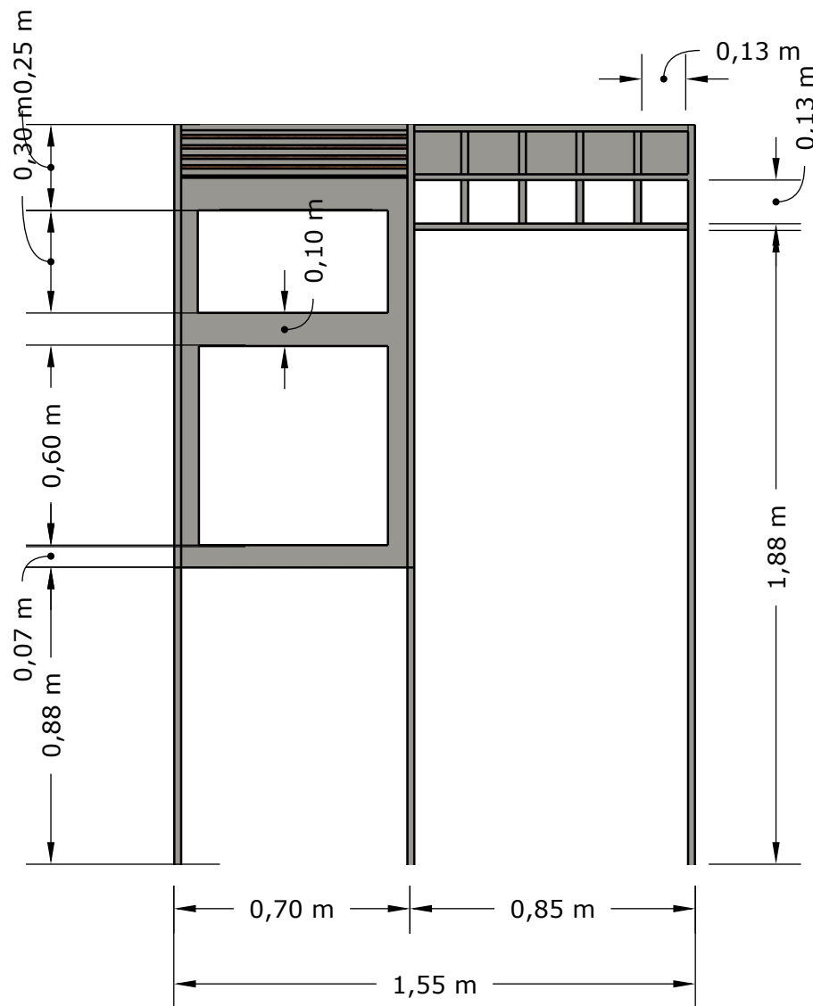
1 VISTA 2 1:20
