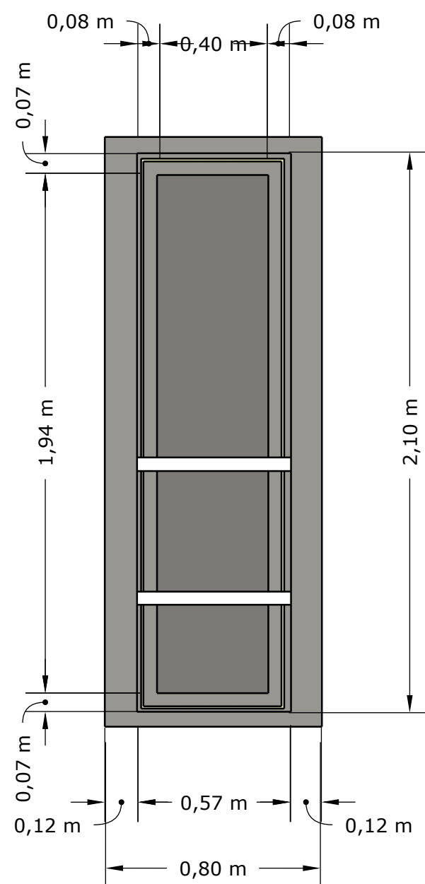
1 VISTA 1 1:20
