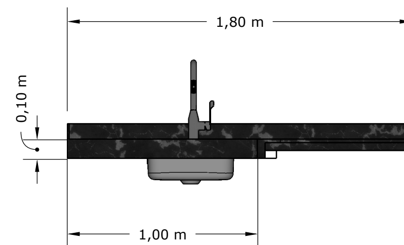
2 VISTA 2 1:20
