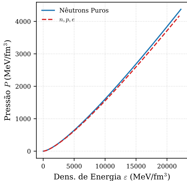
a) Equação de Estado
