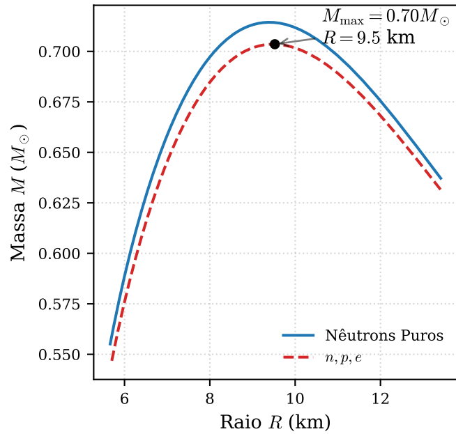
c) Diagrama Massa-Raio
