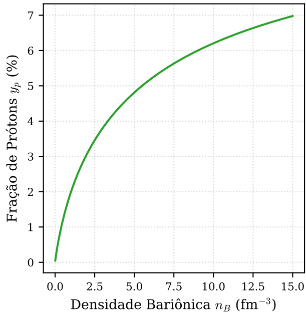
b) Equilíbrio Químico
