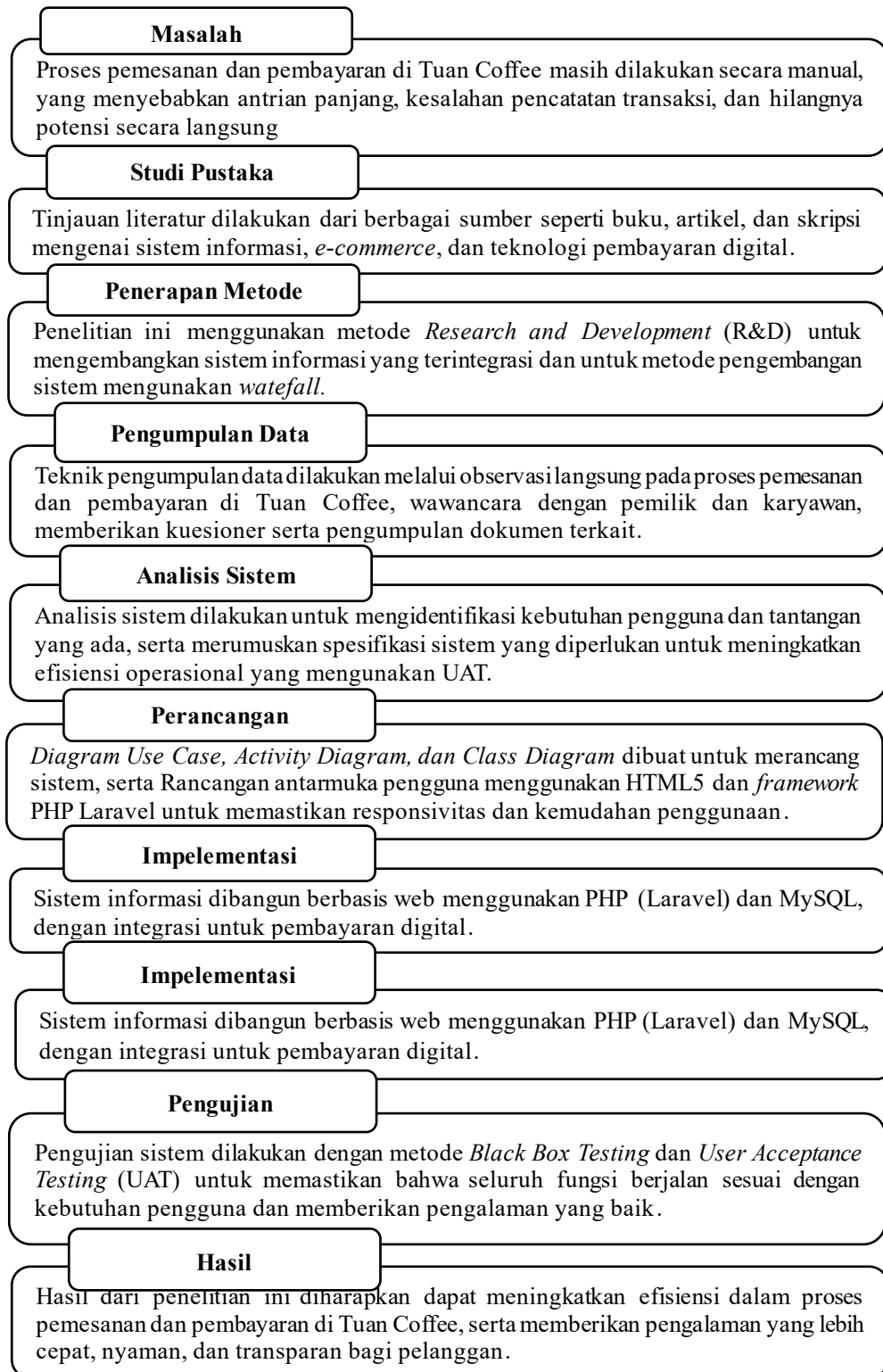
Gambar 2. 3 Kerangka Pemikiran
