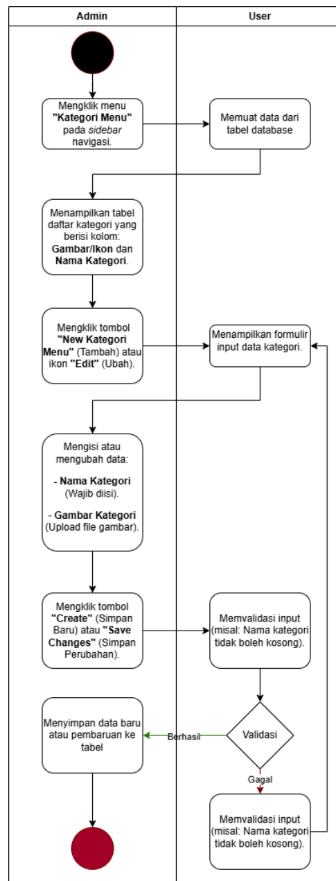
Gambar 4. 9 Activity Diagram Kategori Menu
