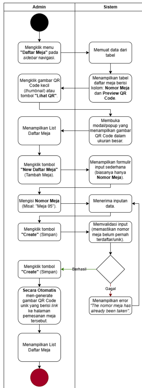
Gambar 4. 6 Activity Diagram Daftar Meja
