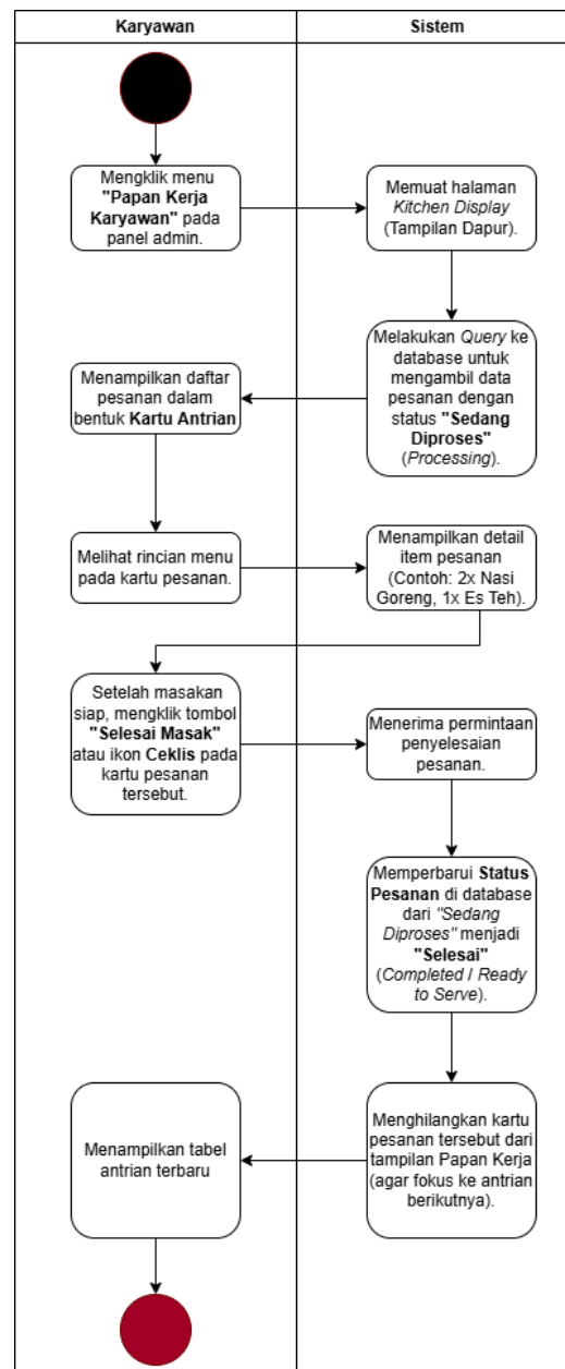
Gambar 4. 11 Activity Diagram Meja Kerja Karyawan
