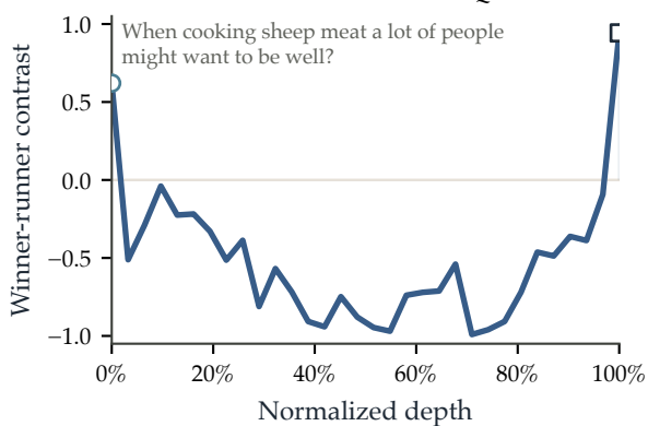
Llama 3.1 8B on CommonsenseQA
