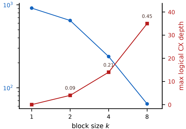
H 4 : trade pays
