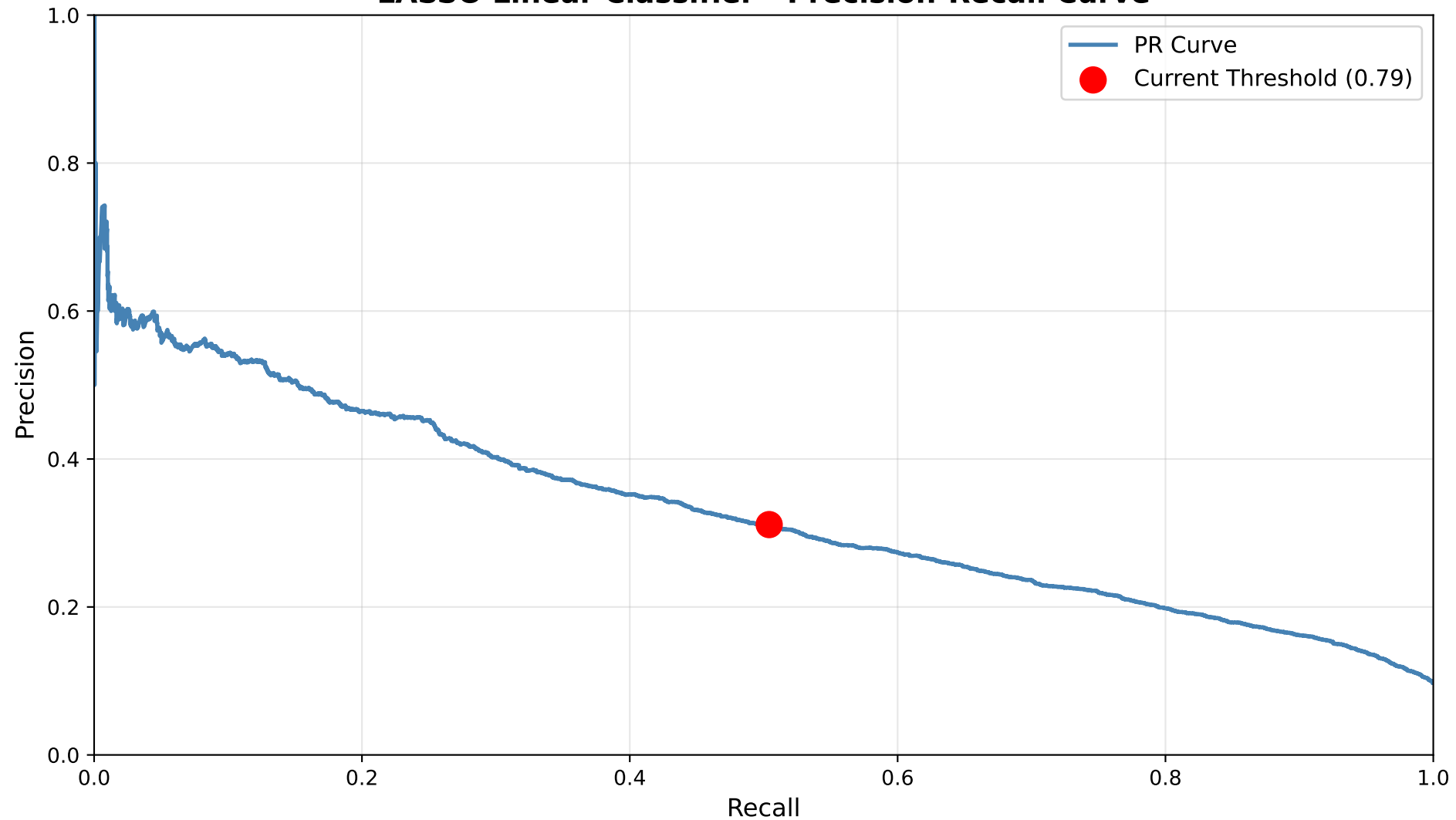
LASSO Linear Classifier - Precision-Recall Curve
