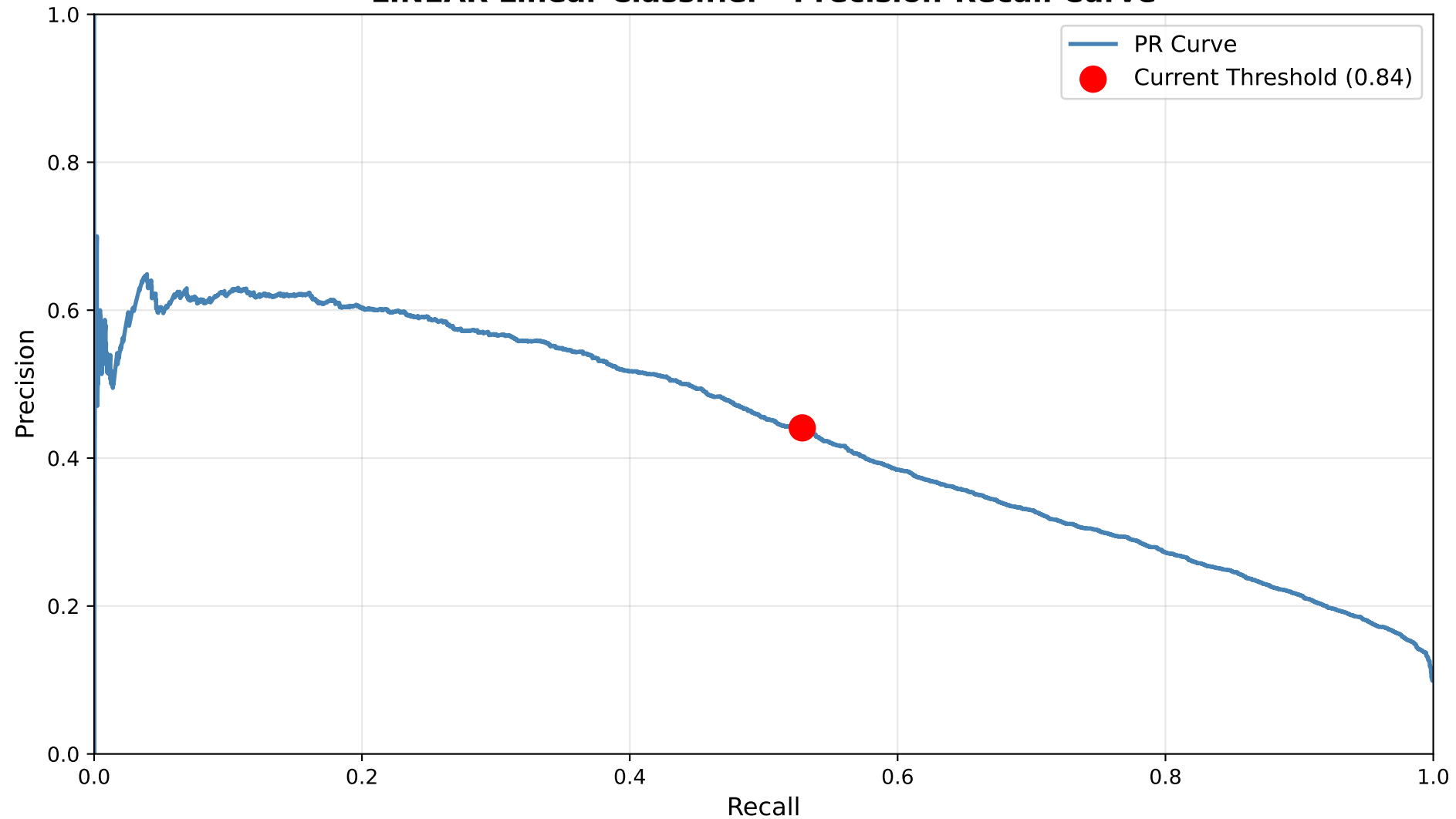
LINEAR Linear Classifier - Precision-Recall Curve
