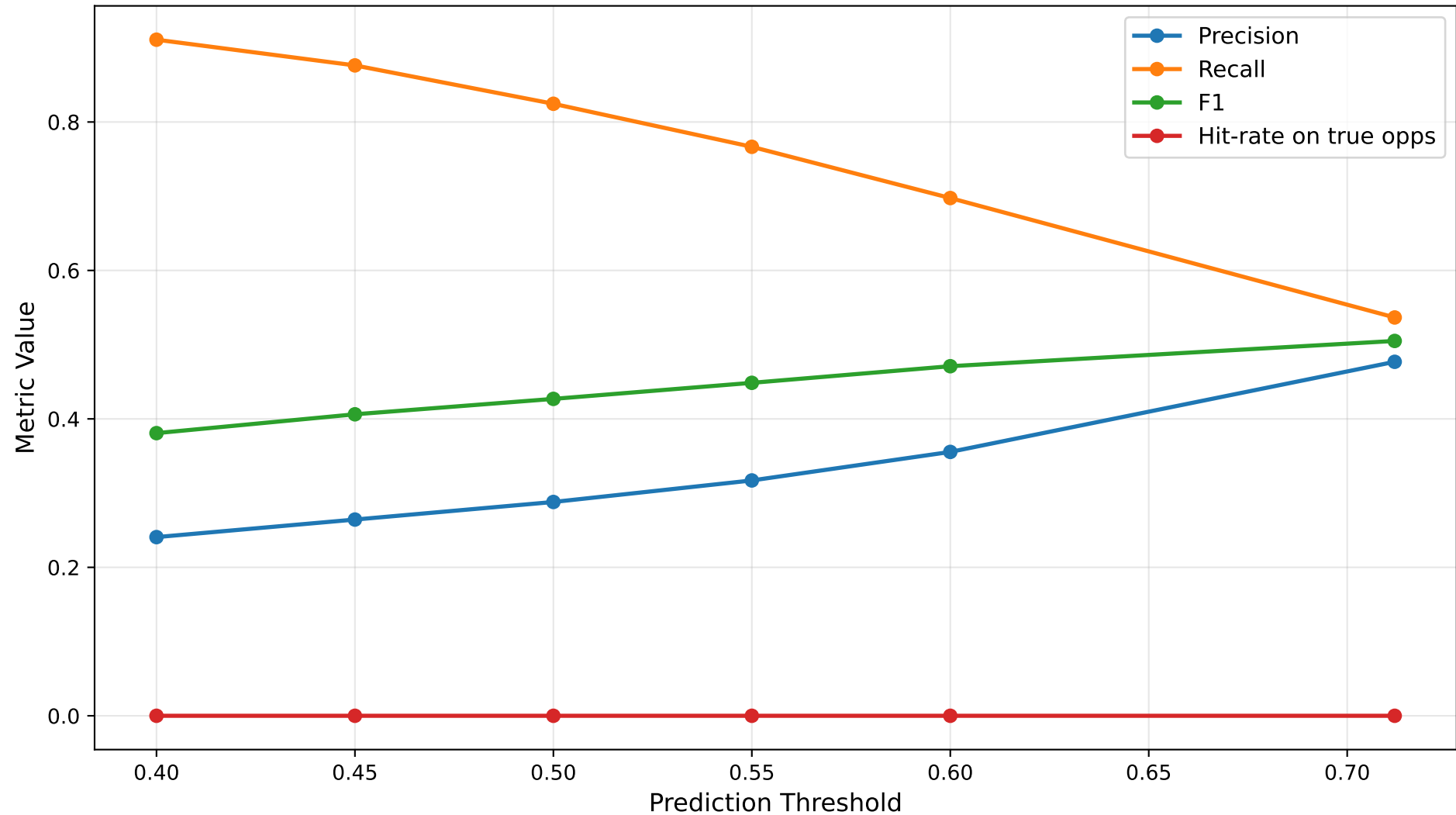
LINEAR Linear Classifier - Threshold Analysis
