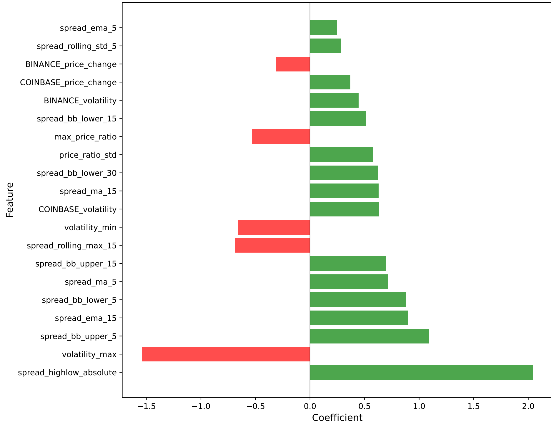
LASSO Linear Classifier - Top 20 Feature Importance
