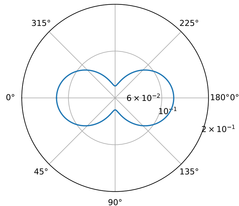
Rayleigh
