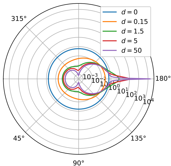
Mie
