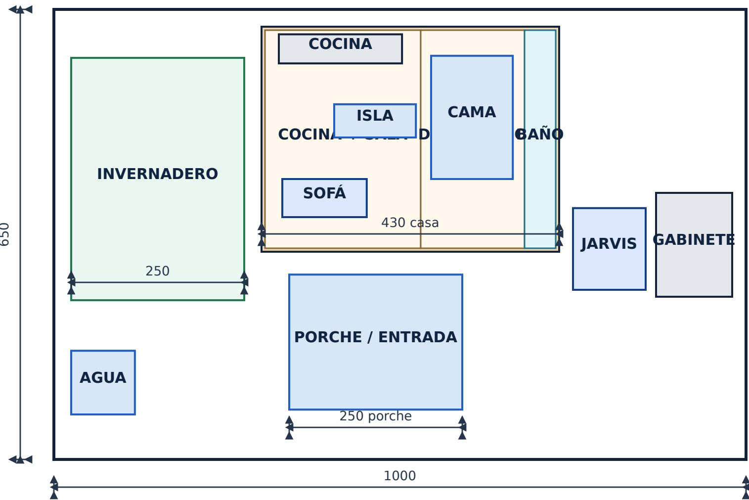
A · PLANTA GENERAL
