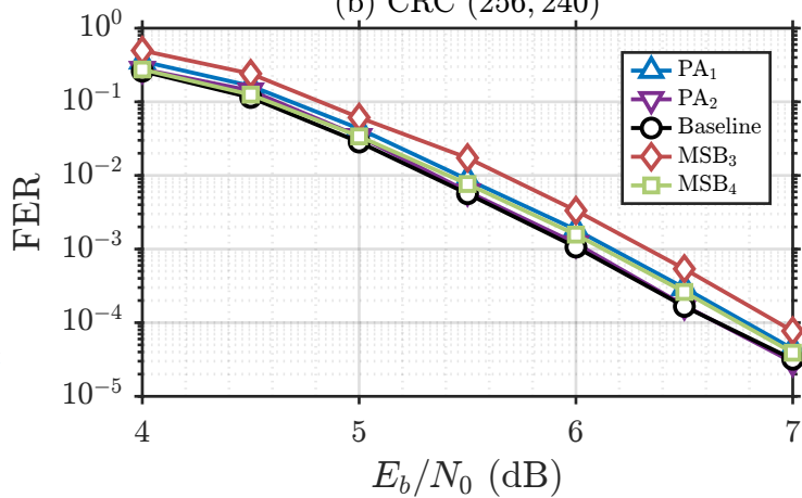
(b) CRC (256, 240)
