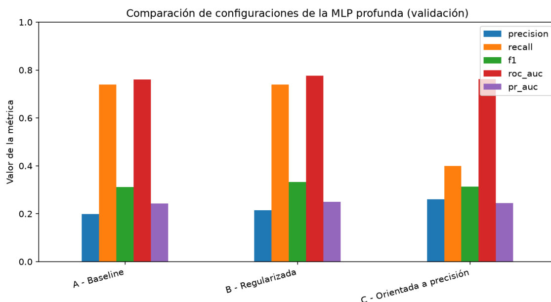
Figura 14. Comparación de las tres configuraciones de la MLP profunda en validación.
