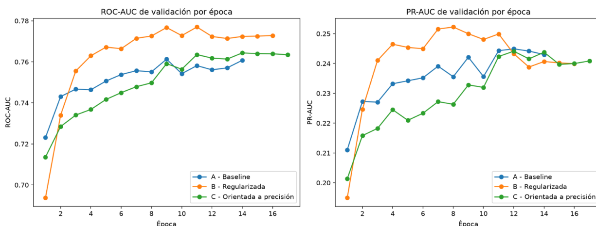
Figura 12. Evolución del ROC-AUC y PR-AUC de validación durante el entrenamiento de las configuraciones MLP.
