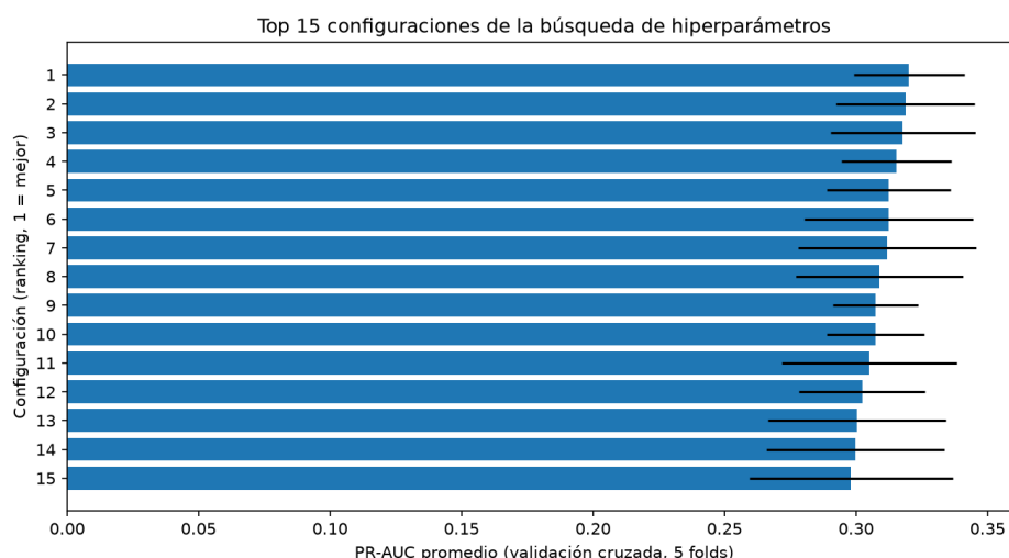
Figura 18. Búsqueda de hiperparámetros de XGBoost (validación cruzada, top 15 configuraciones).
