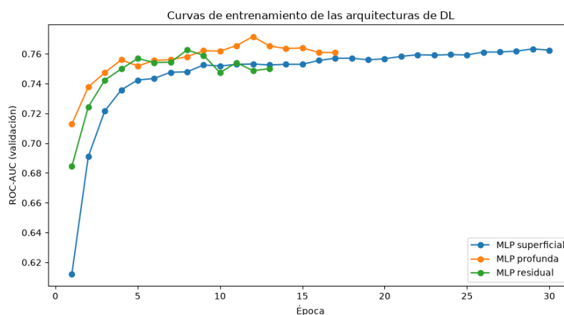
Figura 17. Curvas de entrenamiento de las arquitecturas de deep learning.
