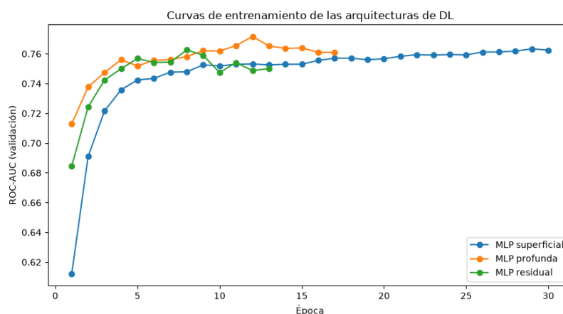
Figura 1. Convergencia de las tres arquitecturas de deep learning en validación
