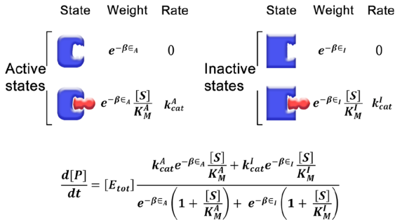
图 2：MWC 模型：状态权重、亲和力和催化速率
