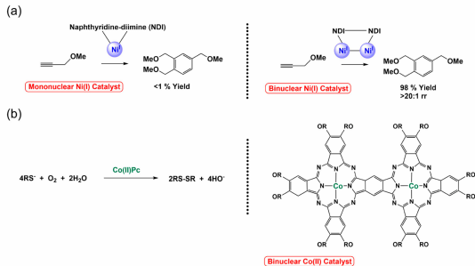
图 27：双核金属催化剂的协同催化
