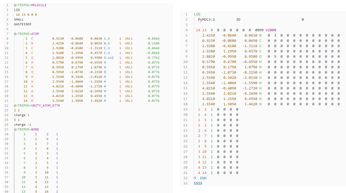
图 16 MOL2 分子结构文件和 SDF 结构数据文件语法高亮演示
