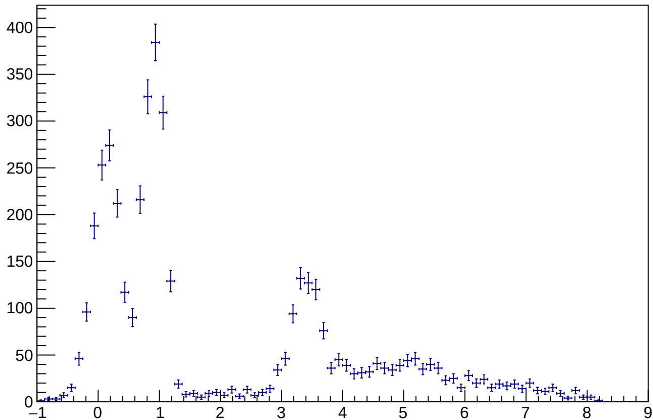
C16(p,d)
