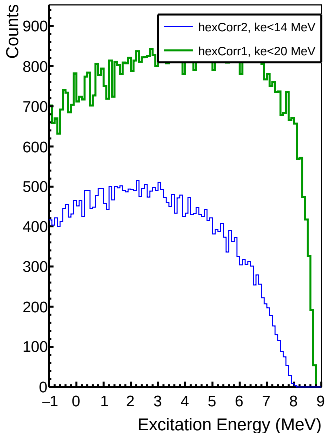
C16(p,d)
