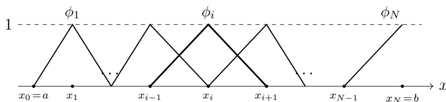
Figura 9.1 Funciones de la base nodal para elementos finitos lineales a trozos ( r = 1 ). Cada \phi_i vale 1 en el nodo x_i y 0 en los demás nodos, y su soporte es [x_{i-1}, x_{i+1}] . En el borde de Neumann x_N = b , la función \phi_N es un “medio sombrero” de soporte [x_{N-1}, x_N] . No hay función de base asociada al nodo x_0 = a debido a la condición de Dirichlet.
