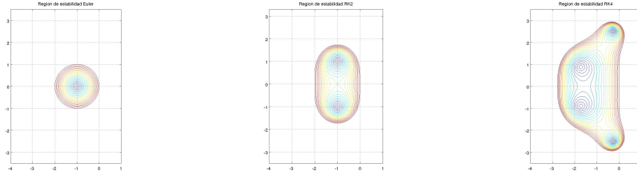
Figura 8.1 Regiones de estabilidad para métodos de Runge-Kutta. Euler o RK1 (izquierda), RK2 (medio), RK4 (derecha).
