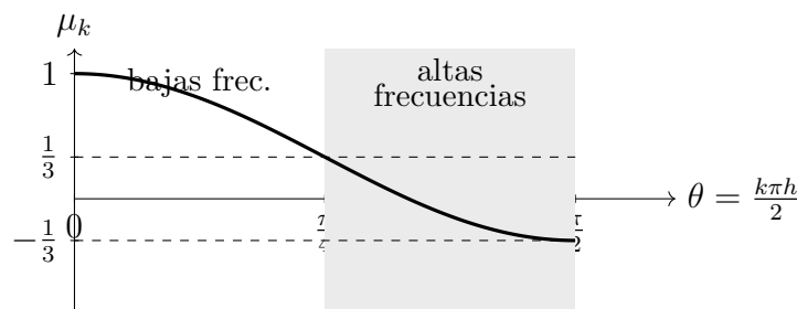
Figura 5.1 Factor de amortiguamiento \mu_k = 1 - 2\omega \sin^2(k\pi h/2) del Jacobi amortiguado con \omega = \frac{2}{3} , en función de la frecuencia \theta = \frac{k\pi h}{2} . En la región de altas frecuencias ( \theta \in [\frac{\pi}{4}, \frac{\pi}{2}] ) se cumple |\mu_k| \leq \frac{1}{3} ; en cambio, los modos suaves ( \theta cerca de 0) tienen \mu_k \approx 1 y casi no se reducen.
