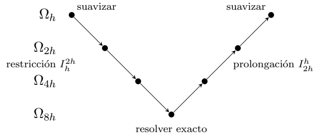
Figura 5.2 Un ciclo en V con cuatro niveles. En la rama descendente se suaviza y se restringe el residuo hacia mallas cada vez más gruesas; en el nivel más grueso se resuelve en forma exacta; en la rama ascendente se prolonga la corrección y se vuelve a suavizar.
