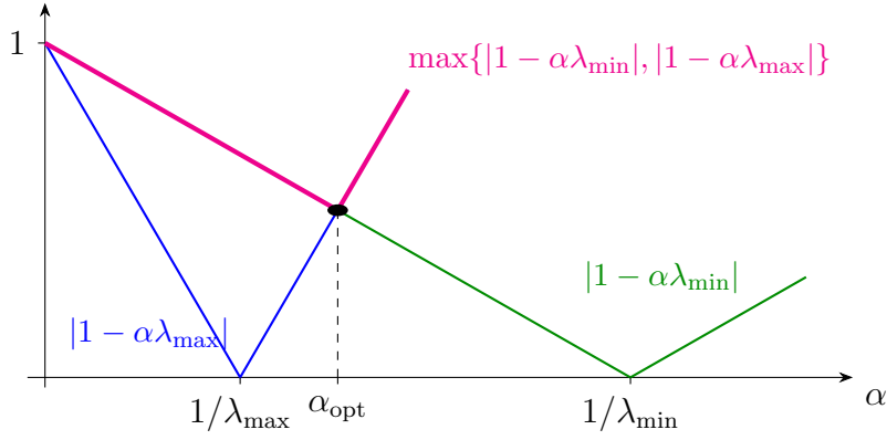
Figura 4.1 Ubicación de \alpha_{\text{opt}} = \operatorname{argmin} \max\{|1 - \alpha\lambda_{\min}|, |1 - \alpha\lambda_{\max}|\} .
