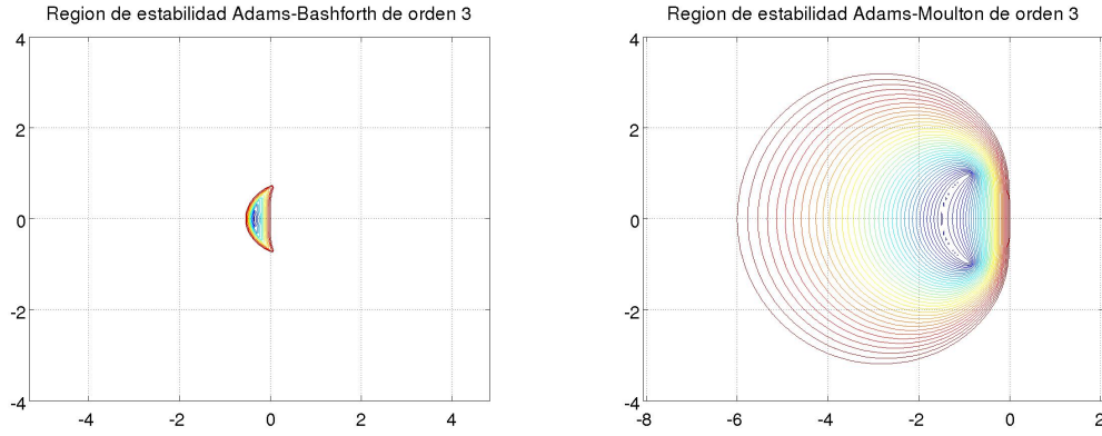
Figura 8.2 Regiones de estabilidad para métodos de Adams-Bashforth (izquierda) y Adams-Moulton (derecha) de orden tres.
