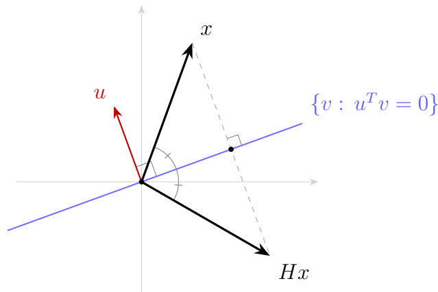
Figura 3.1 La matriz de Householder H = I - uu^T (con \|u\|_2 = \sqrt{2} ) refleja cada vector x respecto del hiperplano \{v : u^T v = 0\} , ortogonal a u : la componente de x en la dirección de u cambia de signo y la componente sobre el hiperplano permanece igual.
