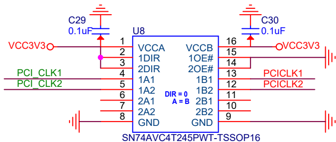
PCI CLOCK 统一 buffer 延时
