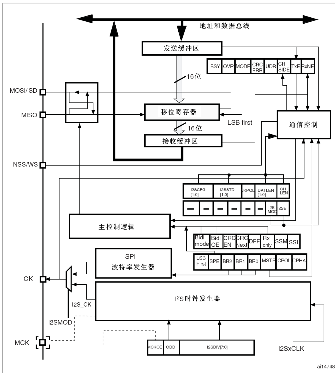
图221 I 2 S框图
