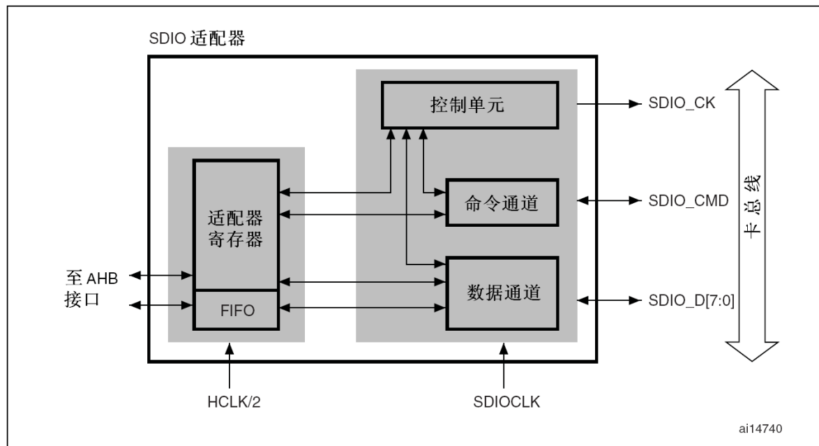
图185 SDIO适配器
