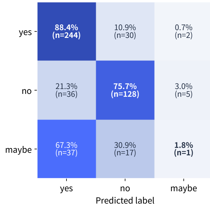
LoRA
