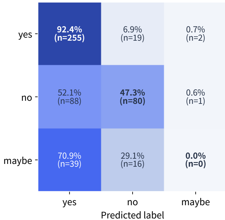
Baseline
