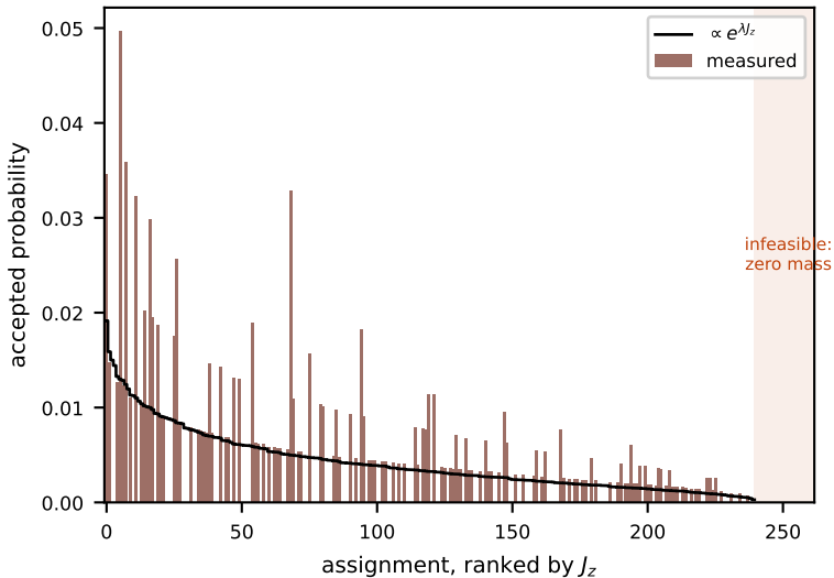
zone Z13: 1 AP, N_z=12 , |\mathcal{F}_z|=240
