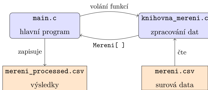
Blokové schéma 1 – procedurální program s datovými soubory (viz Příloha B):
