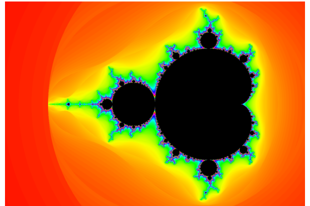
(b) Mandelbrotova množina
