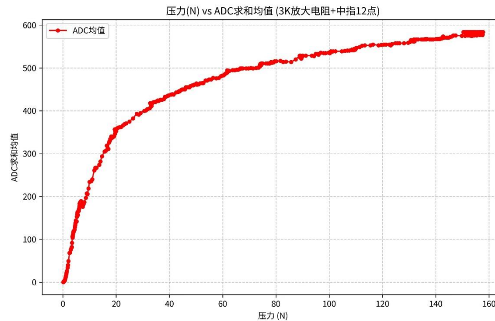
3K放大电阻
