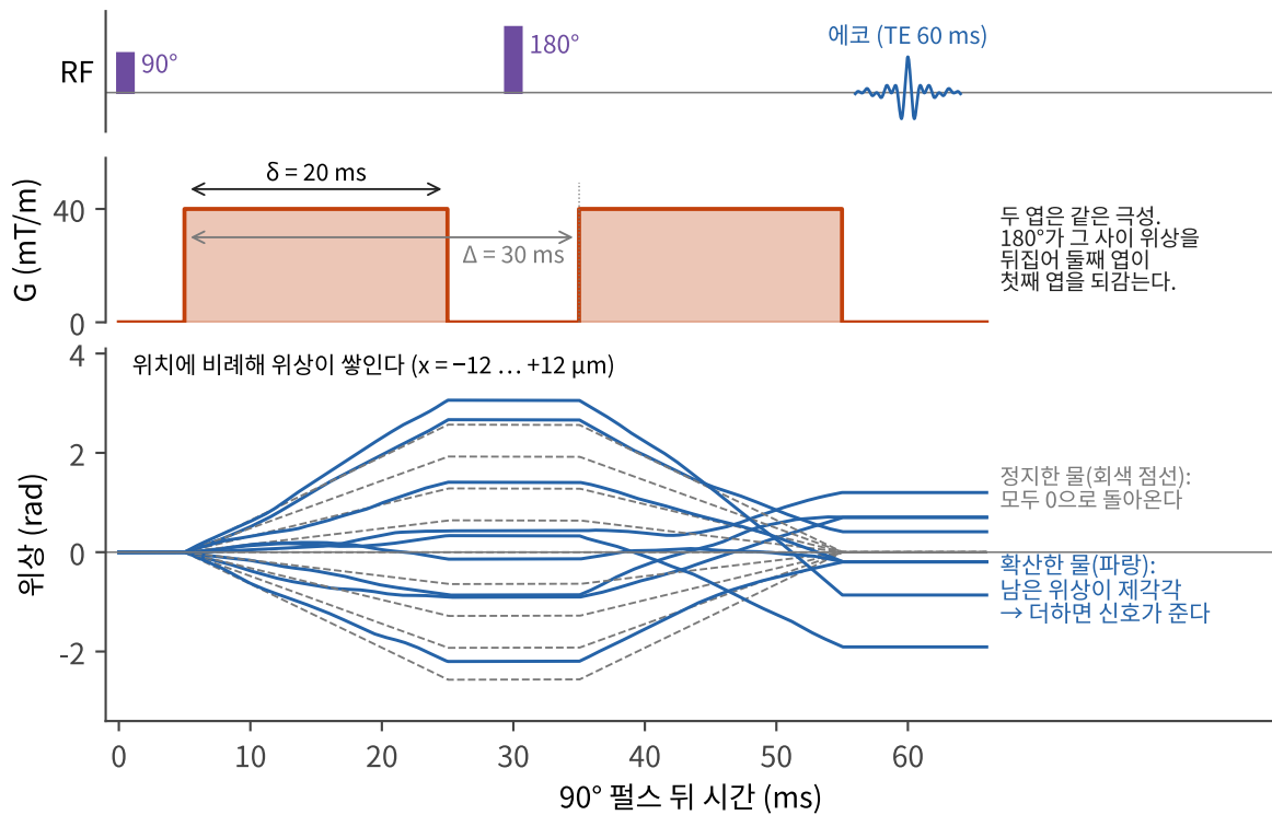
그림 10.3 스테이스칼-태너 펄스 경사 스핀 에코. 180° 펄스 앞뒤에 세기 G = 40 mT/m, 길이 \delta = 20 ms, 간격 \Delta = 30 ms인 경사 엽을 건다. 아래: 위치가 다른 물 분자 9개의 위상(유효 경사로 계산). 정지한 물(화색 점선)은 위치에 비례해 위상이 쌓였다가 모두 0으로 돌아온다. 확산한 물(파랑, D = 1.0 \times 10^{-3} mm 2 /s)은 에코 때 서로 다른 위상이 남는다.
