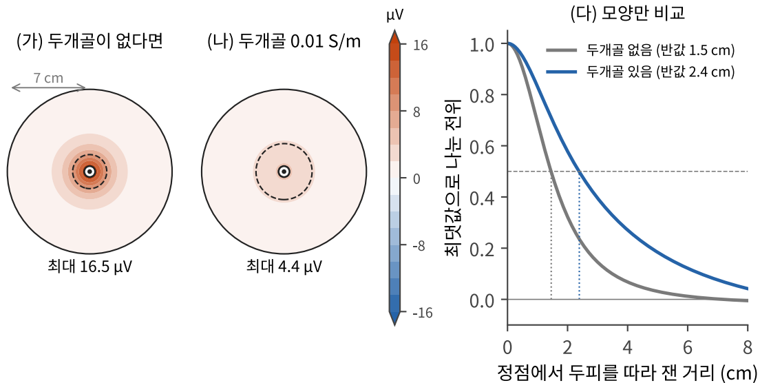
그림 11.2 동심 구 3겹 모형에서 두피 아래 1.7 cm의 지름 방향 쌍극자(10 nA·m)가 만드는 두피 전위. 지도는 정점에서 두피를 따라 7 cm 안쪽을 위에서 본 것이고, 점선은 최대값의 절반 등고선이다. (가) 두개골 전도율이 뇌와 같다고 가정한 경우. (나) 두개골 0.01 S/m. 같은 색 눈금에서 전위가 약 4분의 1로 작아진다. (다) 최대값으로 나누어 모양만 비교하면 두개골이 전위를 1.6배 넓게 번지게 한다.
