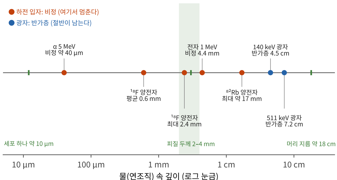
그림 2.6 물(연조직) 속에서 방사선이 들어가는 깊이. 하전 입자(빨강)는 비정에서 멈추고, 광자(파랑)는 반가층마다 절반씩 남으며 멈추지 않는다. 초록 띠는 피질 두께다. α 입자는 세포 몇 개 안에서 멈추고, 양전자는 피질 두께 안팎에서 소멸하며, 영상용 광자는 머리를 빠져나온다.
