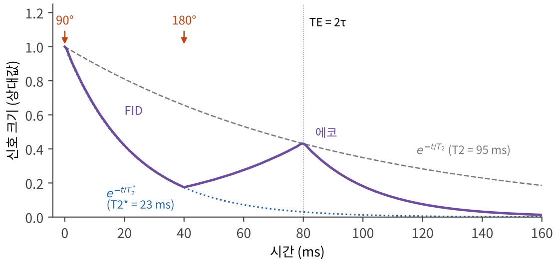
그림 6.4 많은 등색 스핀 묶음을 더해 계산한 FID와 스핀 에코. T_2 = 95 \text{ ms} 에 자기장이 고르지 않은 복셀( T_2' = 30 \text{ ms} )을 가정했다. FID는 T_2^* (약 23 ms)로 빨리 줄지만, 180^\circ 펄스 뒤 위상이 다시 모여 TE = 80 \text{ ms} 에 에코가 생긴다. 에코 꼭짓점은 T_2 곡선(회색 점선) 위에 놓인다.
