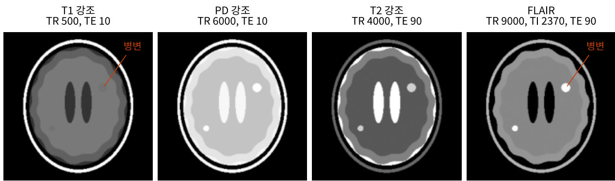
그림 9.4 같은 모형 뇌에 신호 식을 넣어 계산한 네 가지 대비. 오른쪽 위와 왼쪽 아래의 작은 원은 T1과 T2가 길어진 백질 병변이다. T1 강조에서는 거의 보이지 않고, T2 강조에서는 밝지만 뇌척수액과 비슷해 경계가 묻힌다. FLAIR는 뇌척수액을 지워 병변만 밝게 남긴다. 단위는 ms이고, 맨 바깥 고리는 두피 지방이다.
