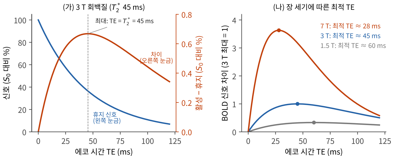
그림 10.1 TE에 따른 BOLD 대비. (가) 3 T 회백질( T_2^* = 45 \text{ ms} )에서 휴지 신호(파랑)와, 활성화로 R_2^* 가 0.4 \text{ s}^{-1} 줄 때의 신호 차이(빨강). 차이는 TE = T_2^* 에서 가장 크다. (나) 장 세기별로 어림한 BOLD 차이(평형 자화 \propto B_0 , \Delta R_2^* 를 1.5 T 0.2, 3 T 0.4, 7 T 1.0 \text{ s}^{-1} 로 잡음). 장이 셀수록 최대값은 커지고 최적 TE는 짧아진다.
