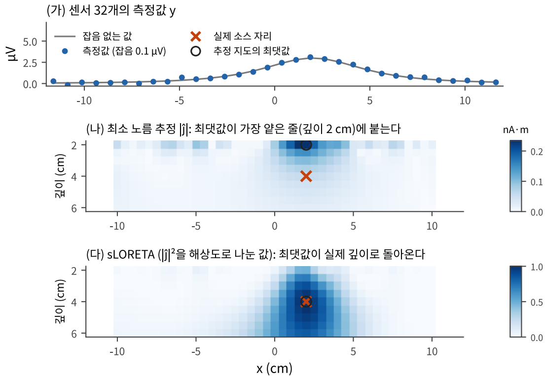
그림 11.7 최소 노름 추정의 깊이 편향. (가) 깊이 4 cm, x = 2 cm에 있는 10 \text{ nA}\cdot\text{m} 쌍극자가 센서 32개에 만든 값과 0.1 \mu V 잡음을 더한 측정값. (나) \lambda^2 = 0.3 의 최소 노름 추정 |j| . 가로 위치는 맞지만 최댓값이 가장 얇은 줄에 붙고, 세기도 실제보다 훨씬 작다. (다) sLORETA처럼 추정값을 해상도로 표준화하면 최댓값이 실제 깊이로 돌아온다. 대신 지도의 퍼짐은 줄지 않는다.
