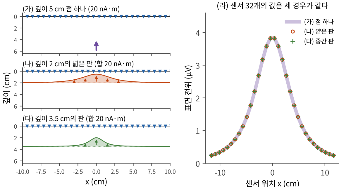
그림 11.5 같은 센서 값을 만드는 세 가지 소스 배치. 반무한 균질 도체에서 (가) 깊이 5 cm의 점 쌍극자 하나, (나) 깊이 2 cm, (다) 깊이 3.5 cm에 펼친 쌍극자 판. 판은 종이 앞뒤로도 펼쳐져 있고, 곡선 높이는 각 판의 면밀도를 그 판의 최댓값으로 나눈 것이다. 판 전체의 쌍극자 합은 셋 모두 20 nA·m다. (라) 센서 32개에서 계산한 전위는 세 경우가 수치 오차(10만분의 1 수준) 안에서 같다.
