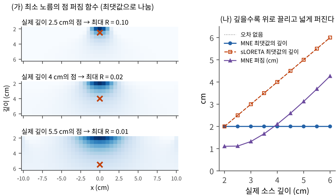
그림 11.8 최소 노름 해상도 행렬의 열(점 퍼짐 함수). (가) x = 0 , 깊이 2.5, 4, 5.5 cm의 단위 점 소스( \times )가 잡음 없는 추정 지도에 그리는 모양을 각자의 최대값으로 나누어 그렸다. 제목의 R 값은 최대값으로, 깊을수록 작아진다. (나) 실제 깊이에 따른 최대값의 깊이와 퍼짐. MNE의 최대값은 늘 가장 얇은 줄에 있고, sLORETA는 실제 깊이를 찾는다. 퍼짐은 깊이와 함께 커진다.
