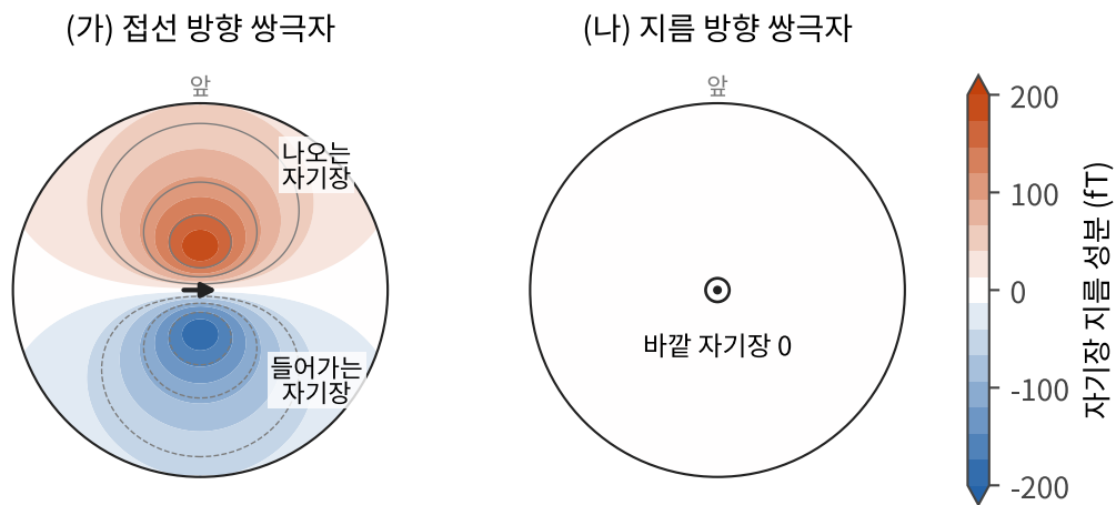
그림 8.3 구형 머리 모형에서 10 \text{ nA} \cdot m 전류 쌍극자가 머리 바깥 센서 구면(반지름 11 cm)에 만드는 자기장의 지름 성분을 정수리 위에서 본 지도. (가) 머리 표면과 나란한 접선 방향 쌍극자는 화살표 양옆으로 나오는 자기장(빨강)과 들어가는 자기장(파랑)의 한 쌍을 만든다. (나) 같은 세기라도 지름 방향을 향한 쌍극자는 머리 바깥에 자기장을 전혀 만들지 않는다.
