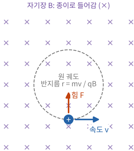
그림 8.4 자기장이 주는 힘. 자기장은 종으로 들어가는 방향(×)이다. (가) 움직이는 양전하는 속도에 수직인 힘을 받아 원 궤도를 돈다. 힘이 늘 속도에 수직이므로 속력은 변하지 않는다. (나) 위로 전류가 흐르는 도선은 왼쪽으로 힘을 받는다. 전동기와 MRI 경사 코일의 진동이 모두 이 힘에서 나온다.
