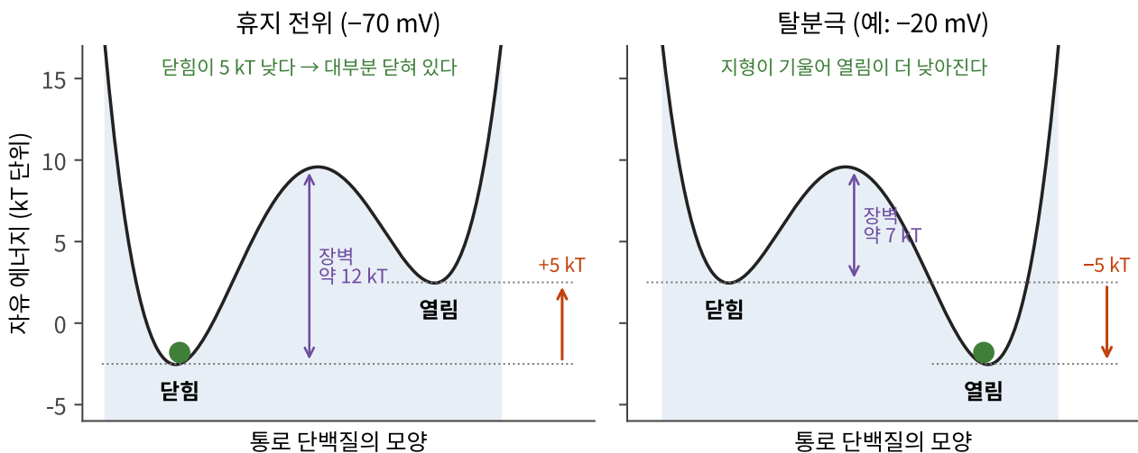
그림 3.6 전압 개폐 통로의 에너지 지형(설명을 위한 단순화). 휴지 전위에서는 닫힌 상태가 5 kT 낮아 통로가 대부분 닫혀 있다. 탈분극하면 지형이 기울어 열린 상태가 더 낮아지고, 닫힘에서 나가는 장벽도 12 kT에서 7 kT로 낮아져 열리는 속도가 약 e^5 \approx 150 배 빨라진다.
