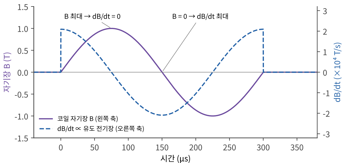
그림 8.7 이상적인 이상성(biphasic) TMS 펄스. 코일 전류와 자기장(보라)이 사인파 한 주기 동안 오르내리고, 유도 전기장은 그 변화를 dB/dt (파랑 점선)을 따른다. 자기장이 최대인 순간에는 유도 전기장이 0이고, 자기장이 0을 지나며 가장 빠르게 변할 때 유도 전기장이 가장 크다. 피질 위치의 최대 자기장을 1 T로 잡았다.
