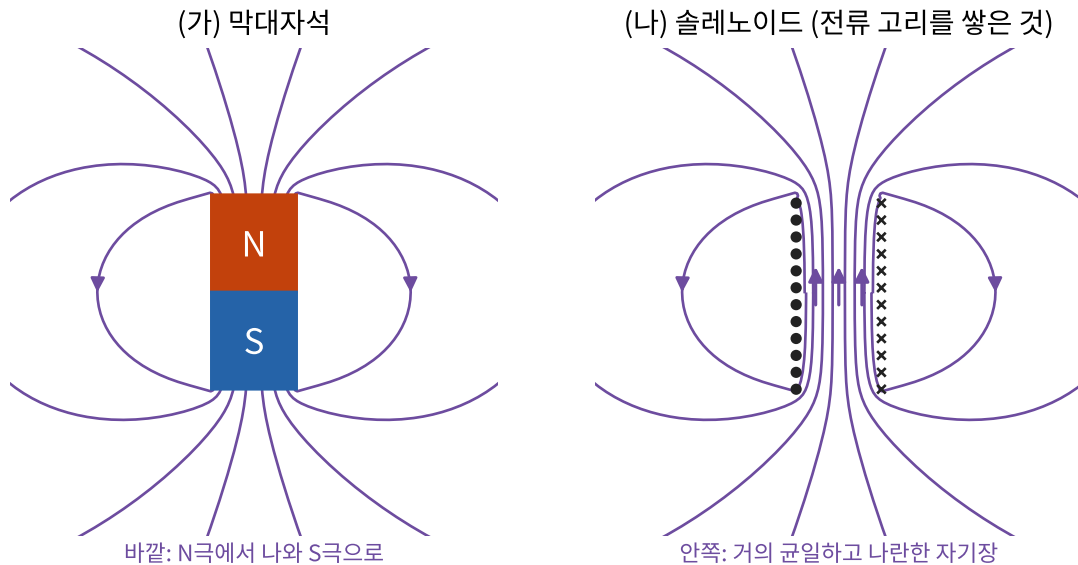
그림 8.1 막대자석과 솔레노이드의 자기력선. 두 그림 모두 같은 솔레노이드(8.2절)의 자기장을 계산해 그렸다. 바깥에서 보면 막대자석과 솔레노이드는 구별되지 않는다. (나)의 ●와 ×는 각각 종이에서 나오고 들어가는 도선이며, 그 안쪽에서 자기장이 거의 균일하다.
