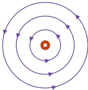
(가) 직선 도선 둘레의 자기장
