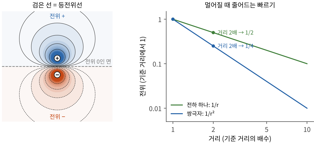
그림 6.5 쌍극자의 전위. 왼쪽: 위쪽 + 주변은 전위가 양(파랑), 아래쪽 - 주변은 음(빨강)이고, 가운데 수평면(점선)은 전위가 0이다. 검은 곡선은 등전위선이다. 오른쪽: 전하 하나의 전위는 거리 2배에 절반이 되지만, 쌍극자의 전위는 4분의 1이 된다. 두 축은 모두 로그 눈금이다.
