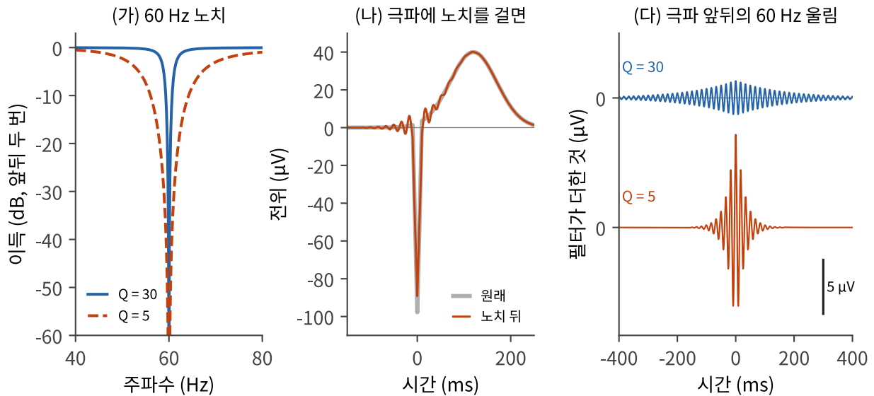
그림 9.4 전원 잡음이 없는 신호에 60 Hz 노치를 걸었다. (가) 앞뒤로 건 노치의 크기 응답. Q = 30 은 폭 2 Hz, Q = 5 는 12 Hz다. (나) 바닥 폭 20 ms, -100 \mu\text{V} 인 극파에 Q = 5 노치를 걸면 파형이 약간 일그러진다. (다) 필터 출력에서 원래 신호를 뺀 것. Q = 30 의 울림은 작지만 수백 ms 이어지고, Q = 5 는 짧지만 크다.
