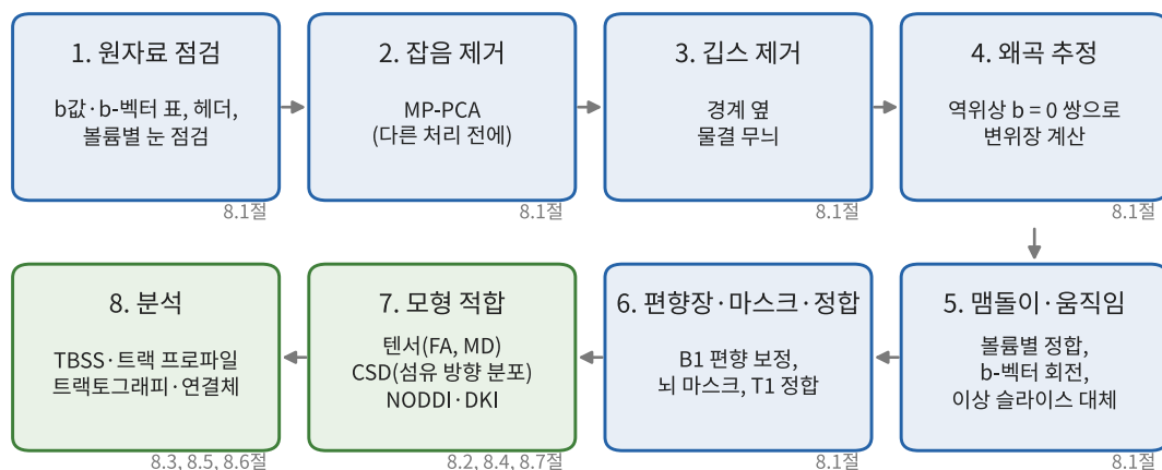
그림 8.1 확산 MRI 분석 파이프라인의 표준 순서. 위 줄(1-4)과 아래 줄의 5-6은 전처리이고, 7-8이 모형 적합과 분석이다. 잡음 제거와 깁스 제거는 보간이 들어가는 보정보다 앞에 둔다. 상자 아래 숫자는 이 장에서 다루는 절이다.
