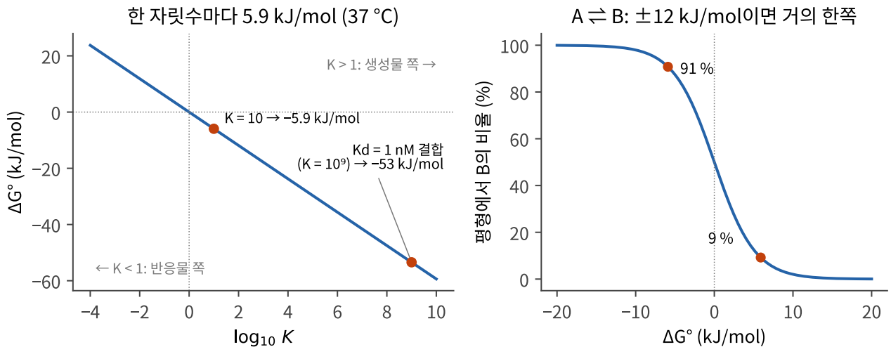
그림 6.2 표준 자유에너지와 평형 상수(37 °C). 왼쪽: \Delta G^\circ 는 \log_{10} K 에 정비례하며, 한 자릿수마다 5.9 kJ/mol씩 바뀐다. K_d = 1 \text{ nM} 인 결합은 약 -53 kJ/mol에 해당한다. 오른쪽: A \rightleftharpoons B 평형에서 B의 비율은 \Delta G^\circ 약 \pm 12 \text{ kJ/mol} 안에서만 크게 바뀌고, 그 바깥에서는 거의 한쪽으로 쏠린다.
