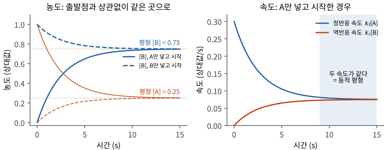
그림 6.1 A \rightleftharpoons B 반응(정반응 속도 상수 0.3/s , 역반응 0.1/s )이 평형에 다가가는 모습. 왼쪽: A만 넣고 시작하든(실선) B만 넣고 시작하든(점선) 같은 평형 농도(B 75 %, A 25 %)에 이른다. 오른쪽: A만 넣고 시작하면 정반응 속도는 줄고 역반응 속도는 늘어 결국 같아진다. 농도가 멈춘 뒤에도 두 반응은 계속 일어난다.
