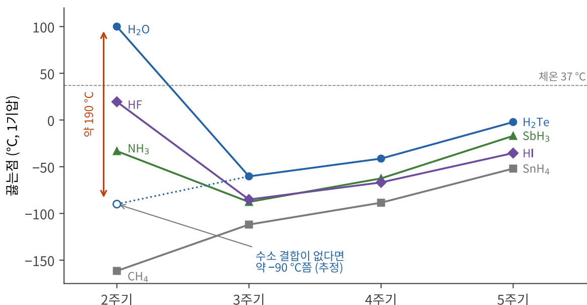
그림 3.3 같은 족 수소 화합물의 끓는점. 아래 주기로 갈수록 분자가 커져 분산력이 세지므로 끓는점이 오른다(14족, 회색). 수소 결합을 하는 \text{H}_2\text{O} , \text{HF} , \text{NH}_3 만 2주기에서 크게 뛰어 오른다. 물은 추세로 예상되는 값(빈 원)보다 약 190^\circ\text{C} 높은 온도에서 끓는다.
