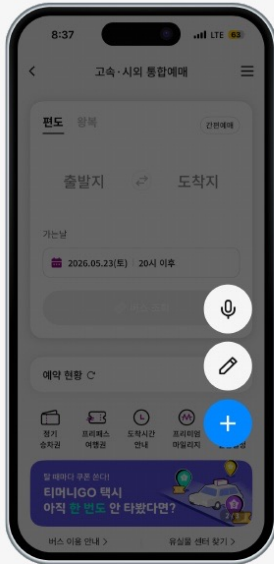
기존 화면
