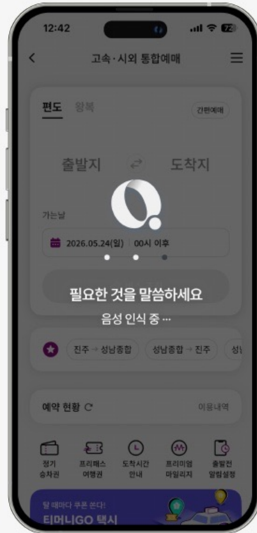
음성 인식
