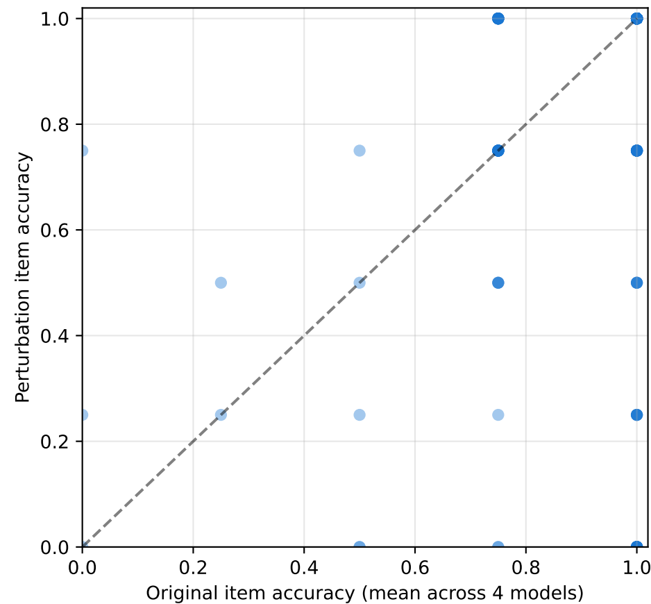
GSM8K r = 0.273 , shift = +0.134
