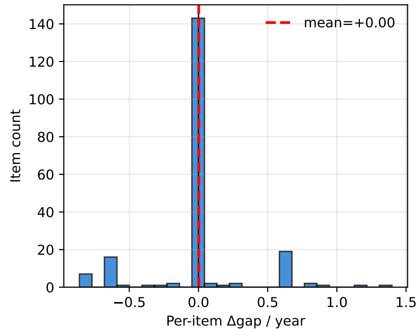
GSM8K
