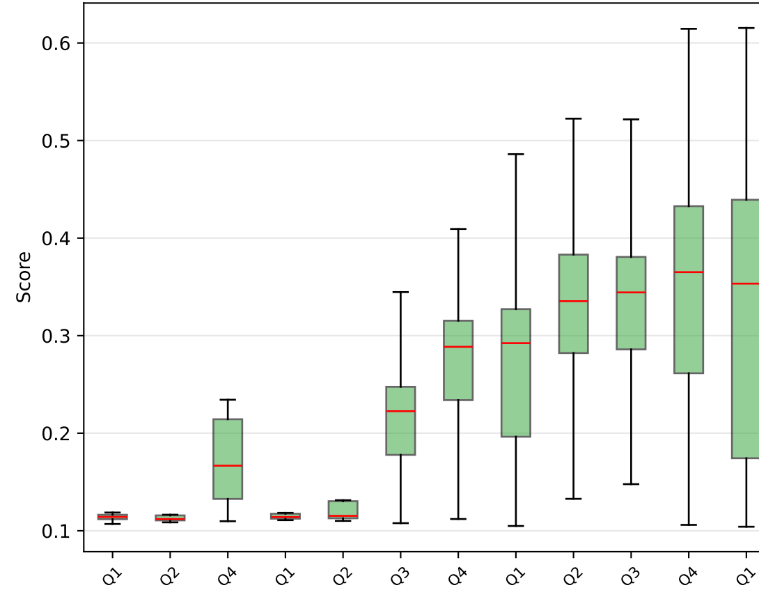
MATH Lvl5
