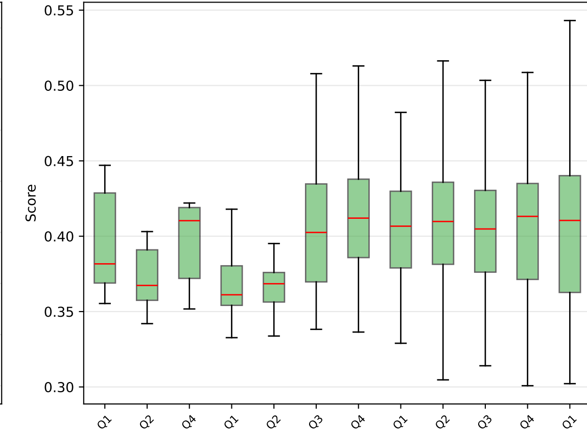
MUSR
