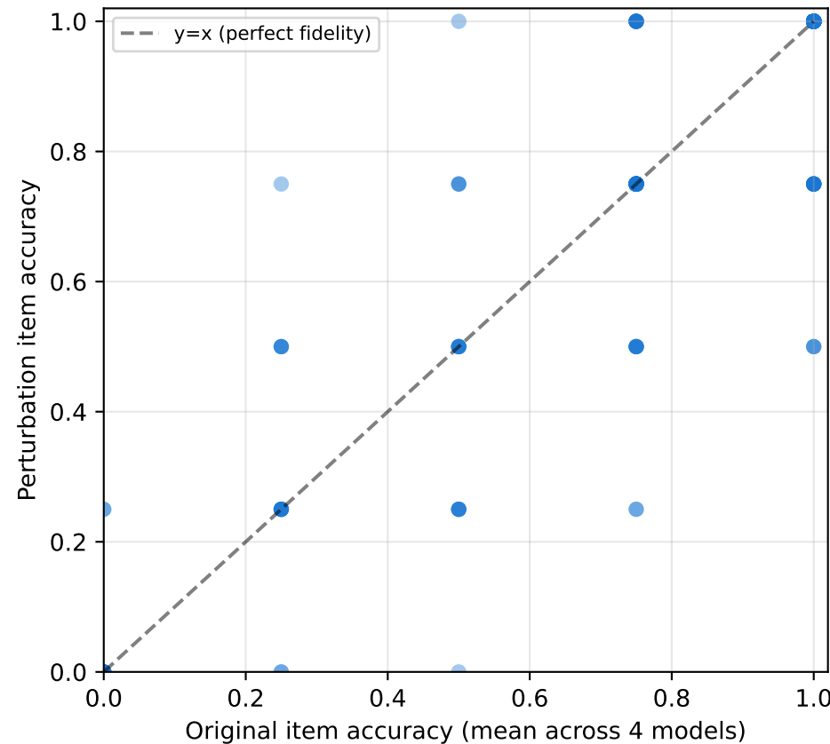
MMLU
