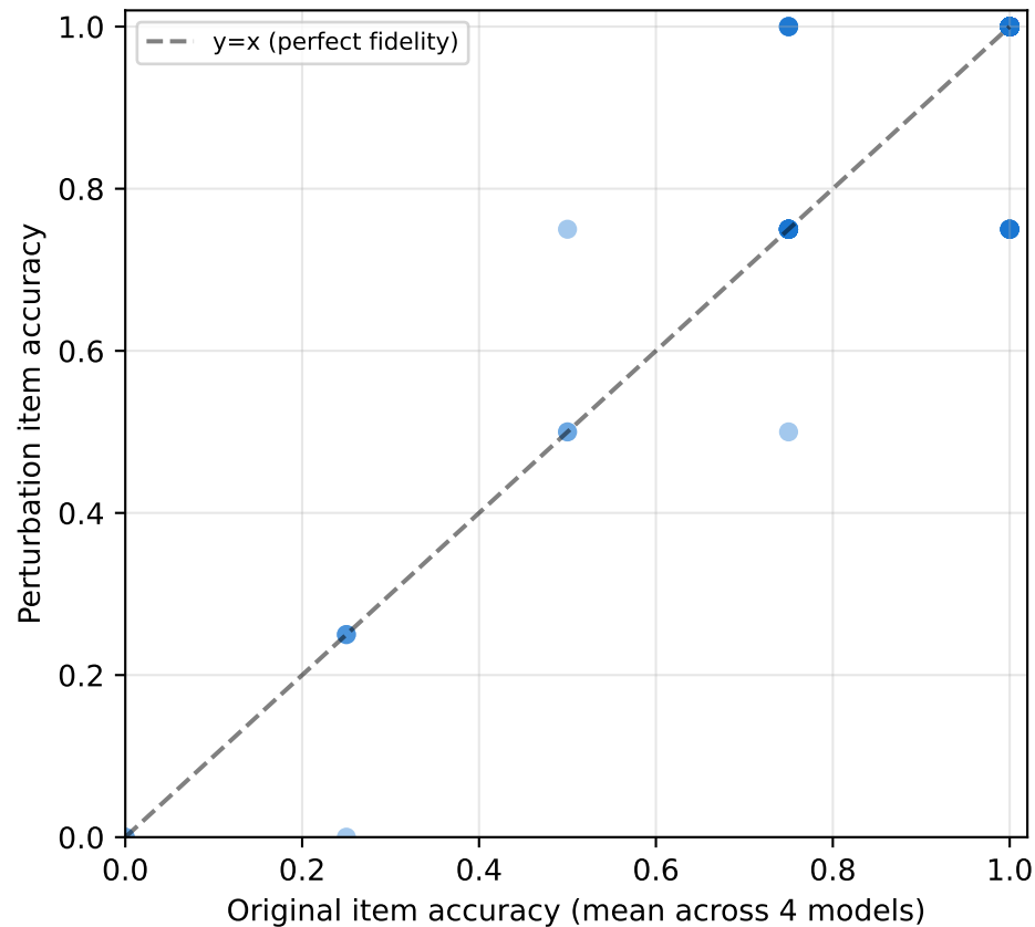
ARC
