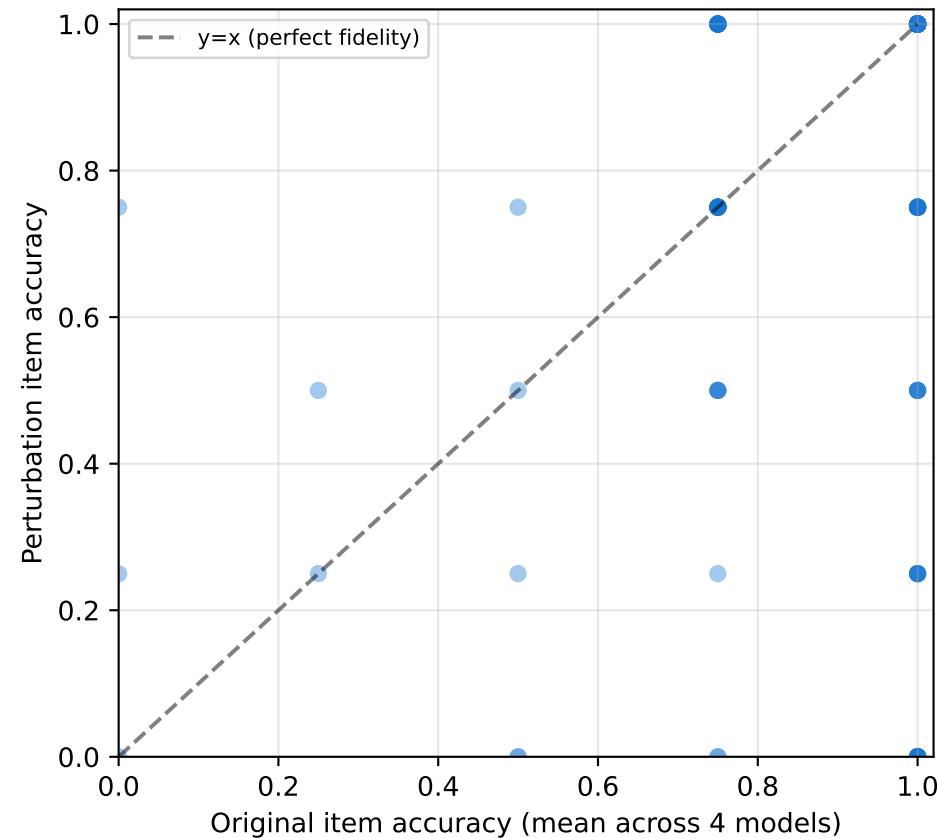
GSM8K
