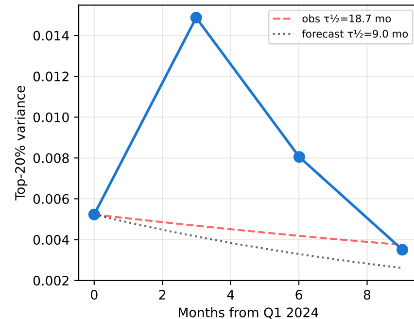
BBH
