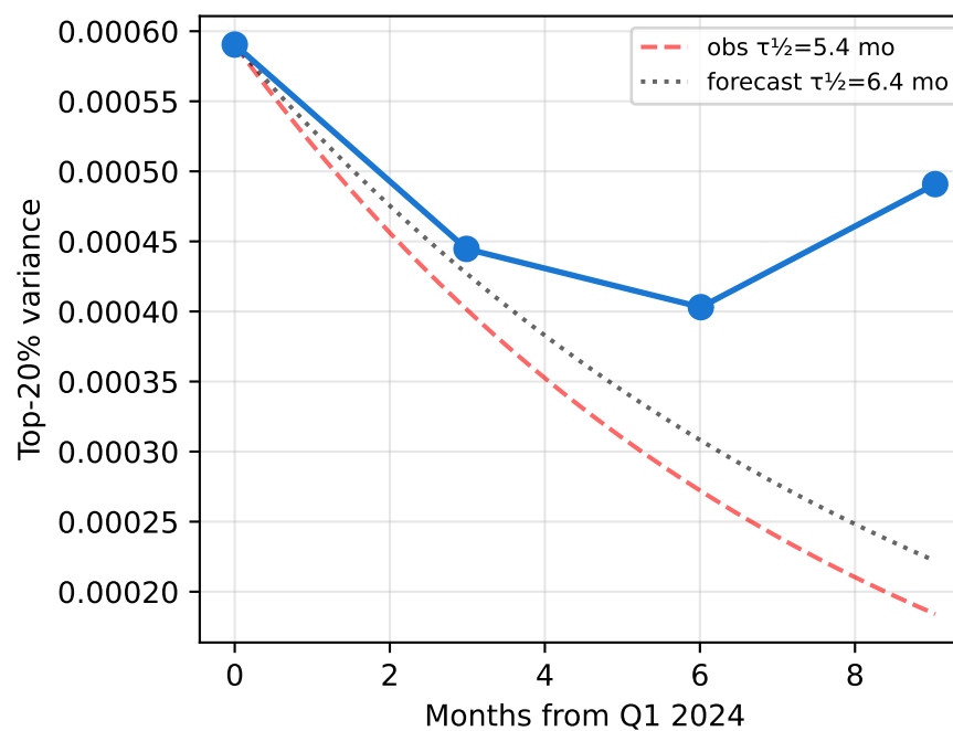
MUSR
