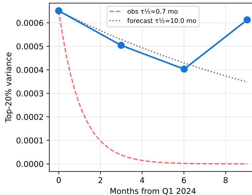
MUSR
